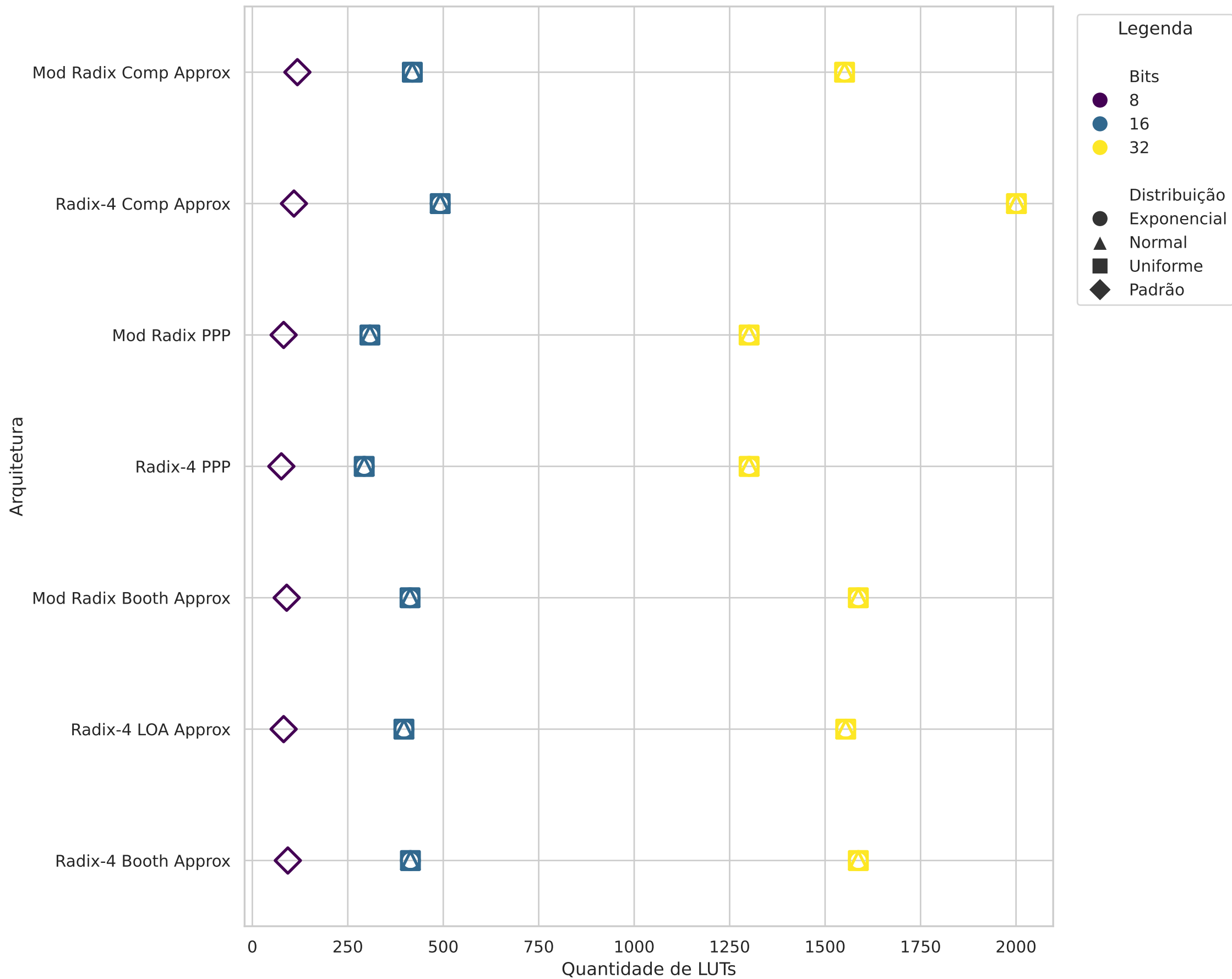
Comparação de Uso de LUTs - Aproximados
