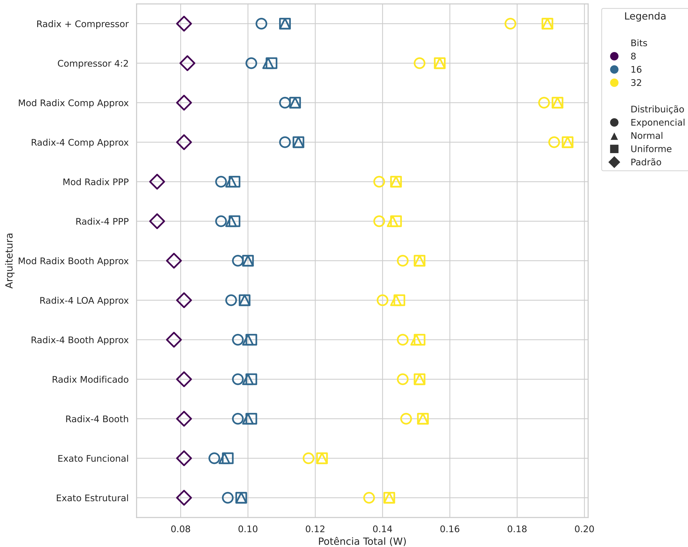
Comparação de Potência Total - Todos
