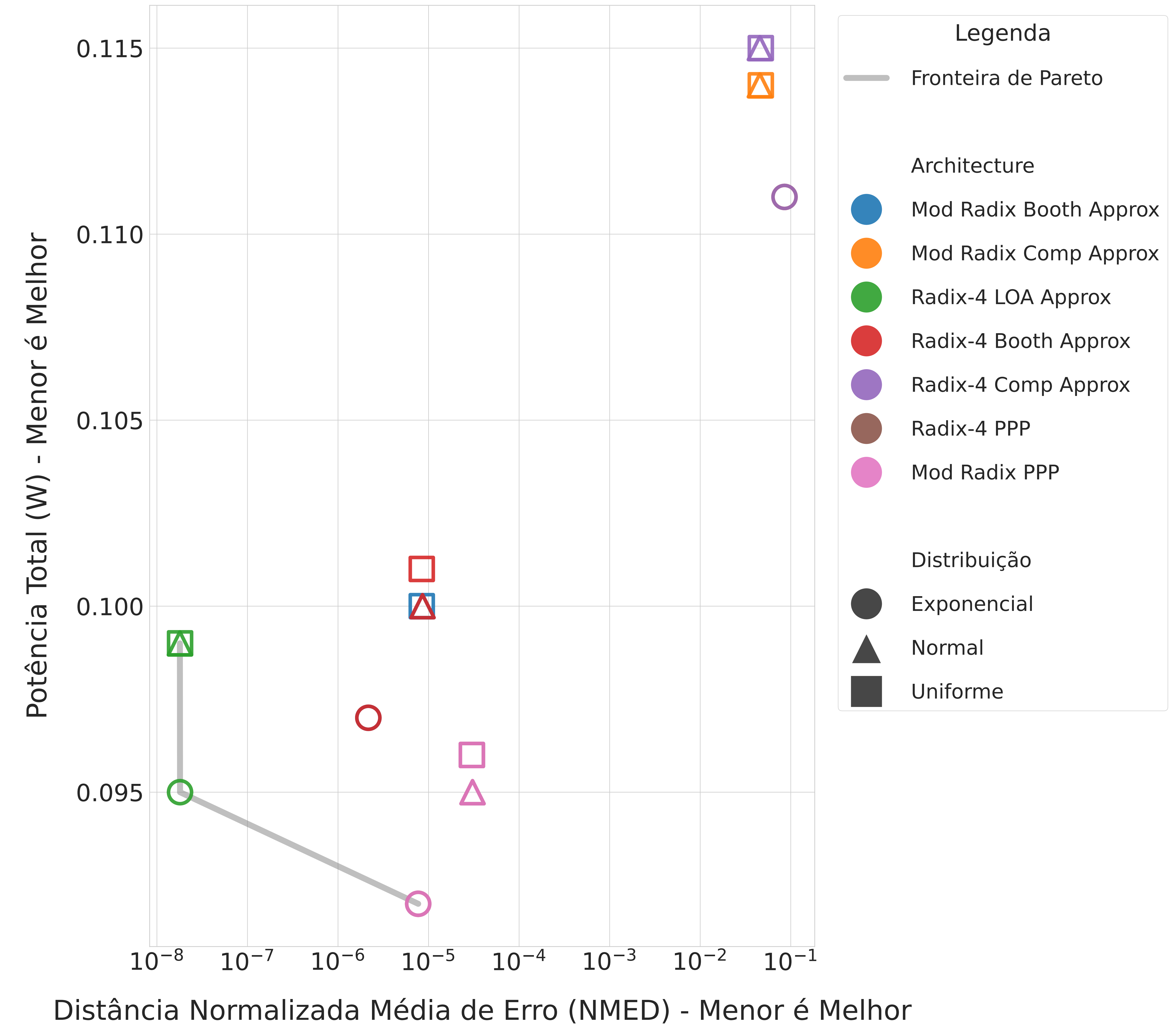
Trade-off: Potência Total (W) vs Erro Normalizado (NMED) - 16 Bits
