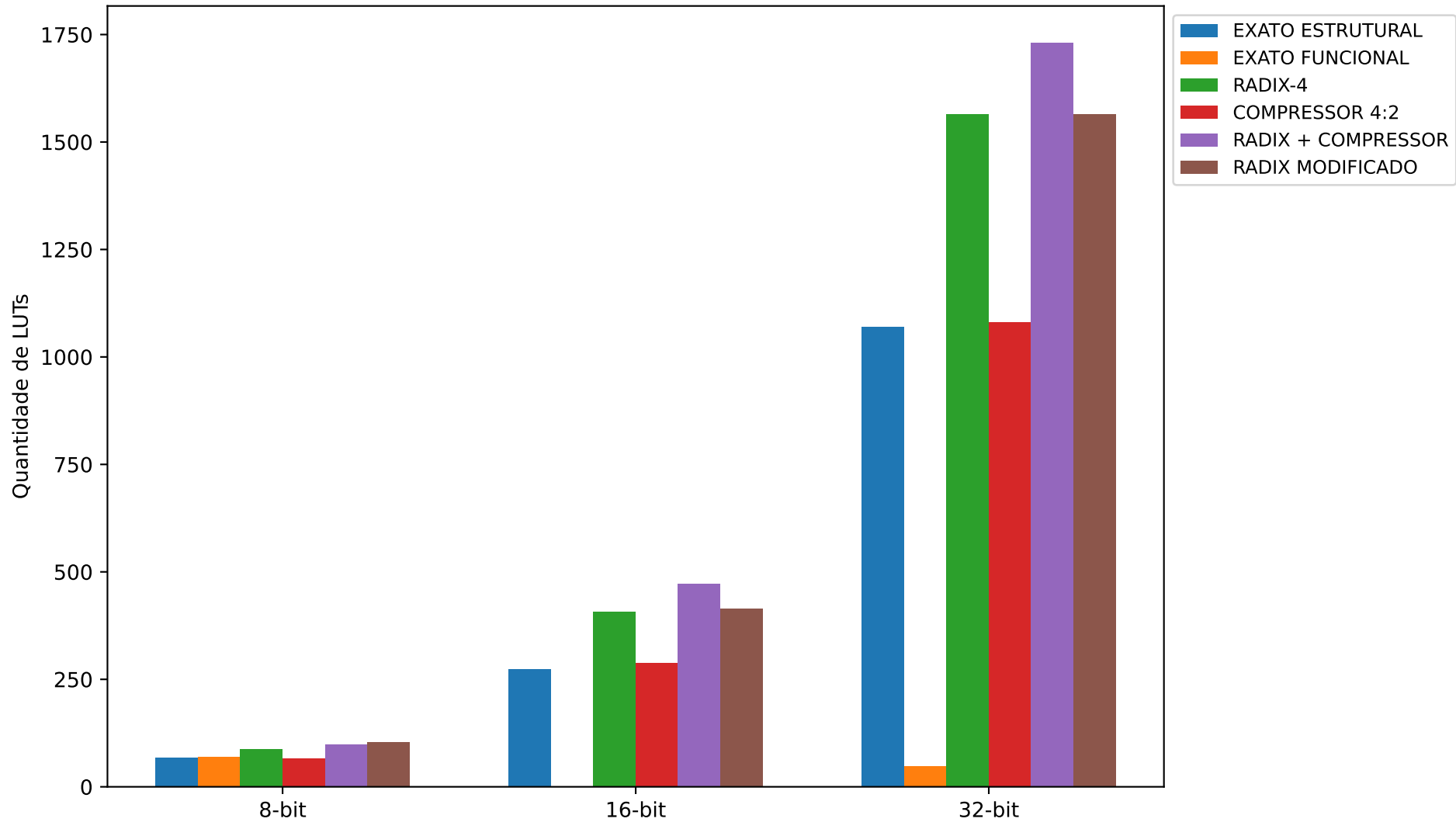
Comparação de uso de LUTs
