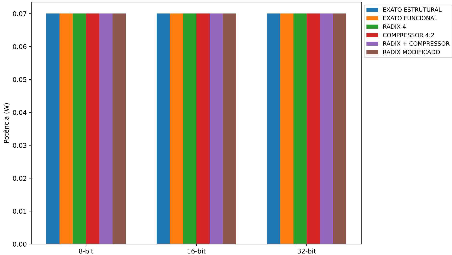
Comparação de Potência Estática
