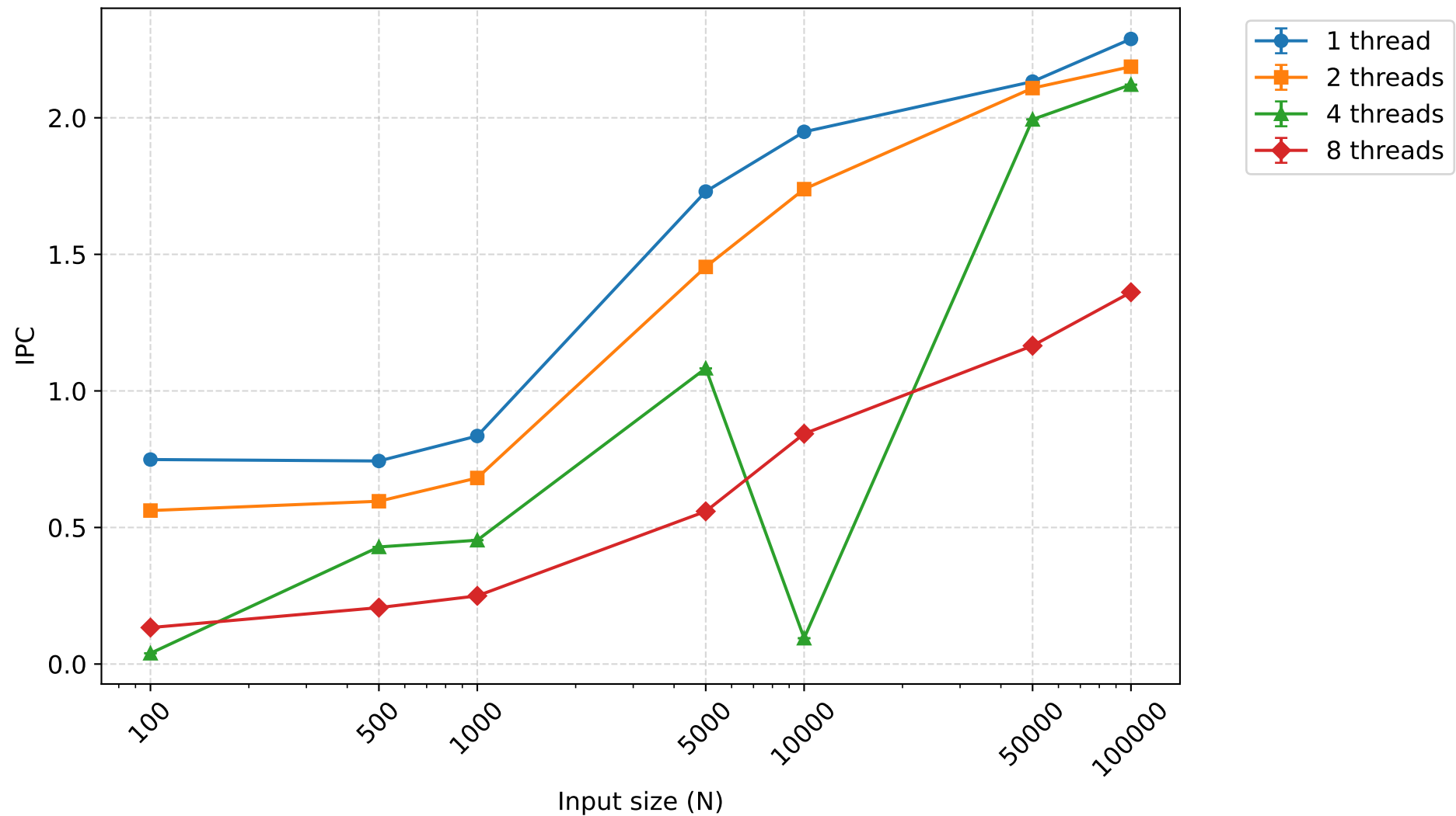
IPC - bitonicsort (mean \pm 95% CI)
