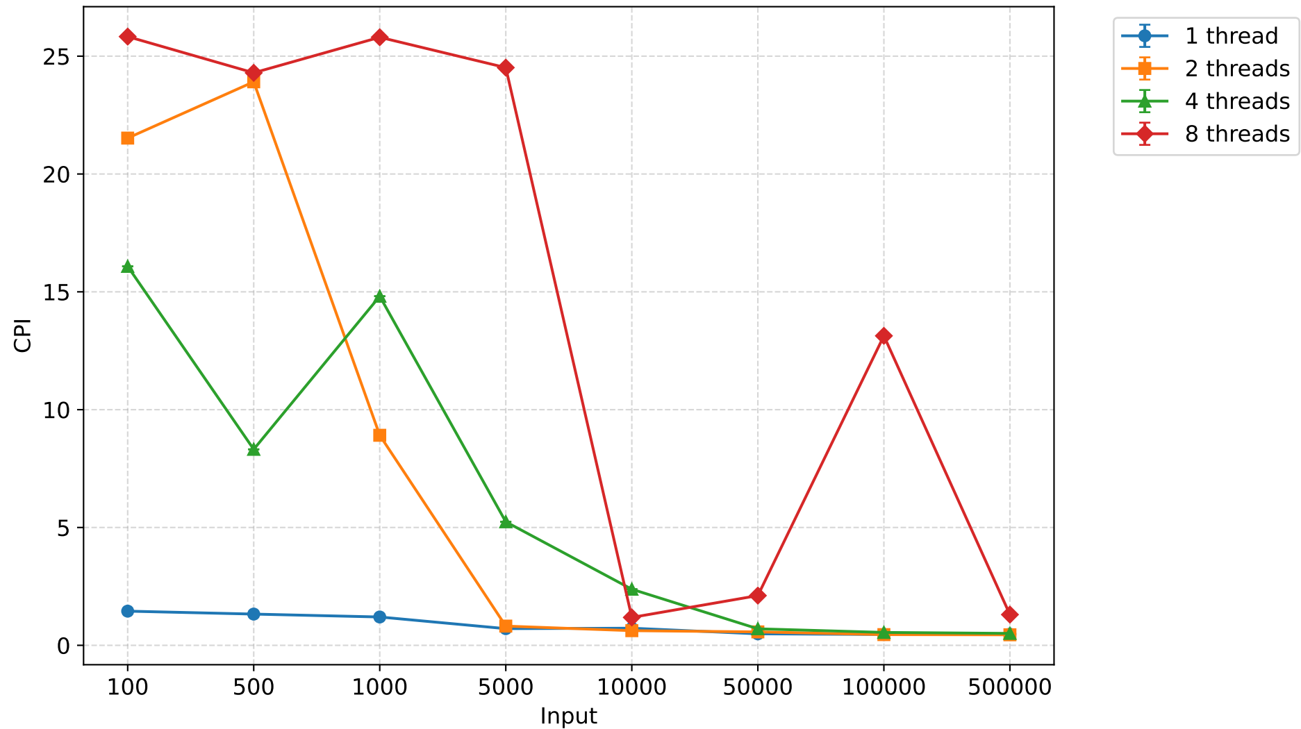
CPI - bitonicsort (mean \pm 95% CI)
