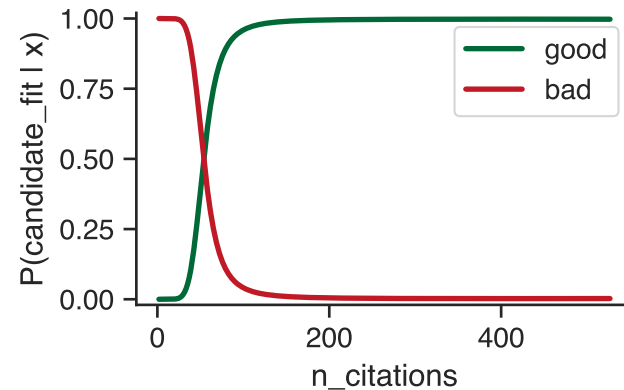
B) Posterior (1D)
