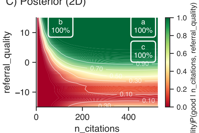
C) Posterior (2D)
