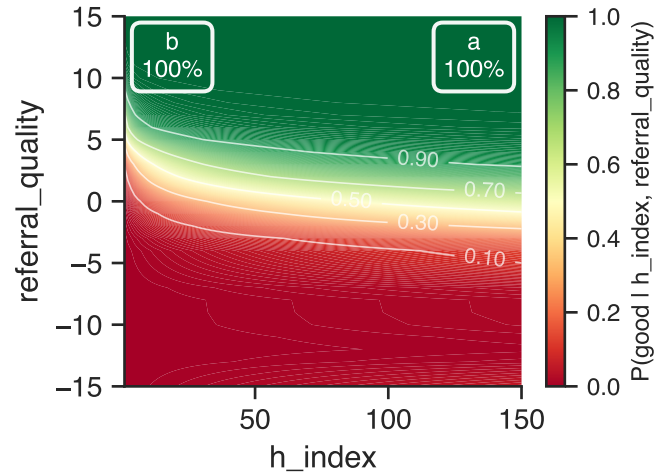
C) Posterior (2D)
