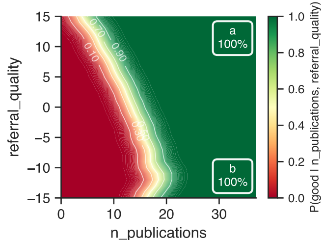
C) Posterior (2D)
