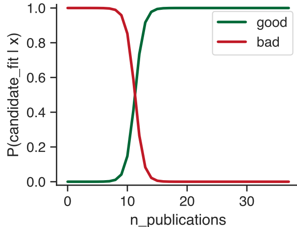
B) Posterior (1D)
