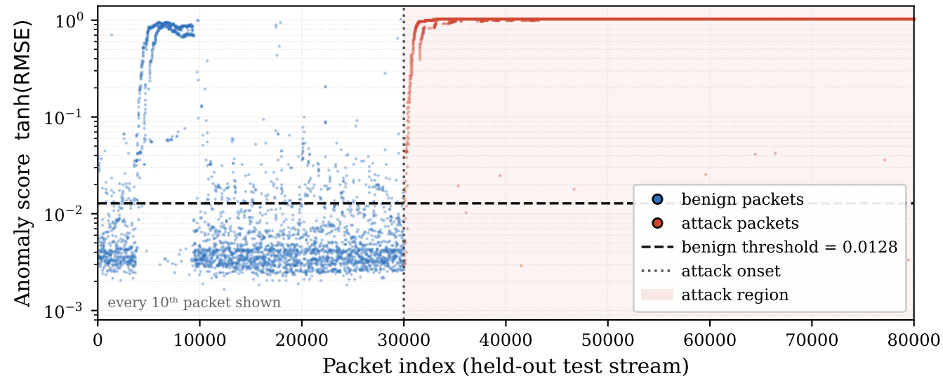
Kitsune (per-packet RMSE) — DoS SYN Flood (CICIoT2023)
