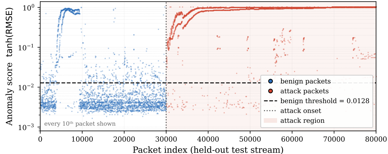
Kitsune (per-packet RMSE) — MITM ARP Spoofing (CICIoT2023)
