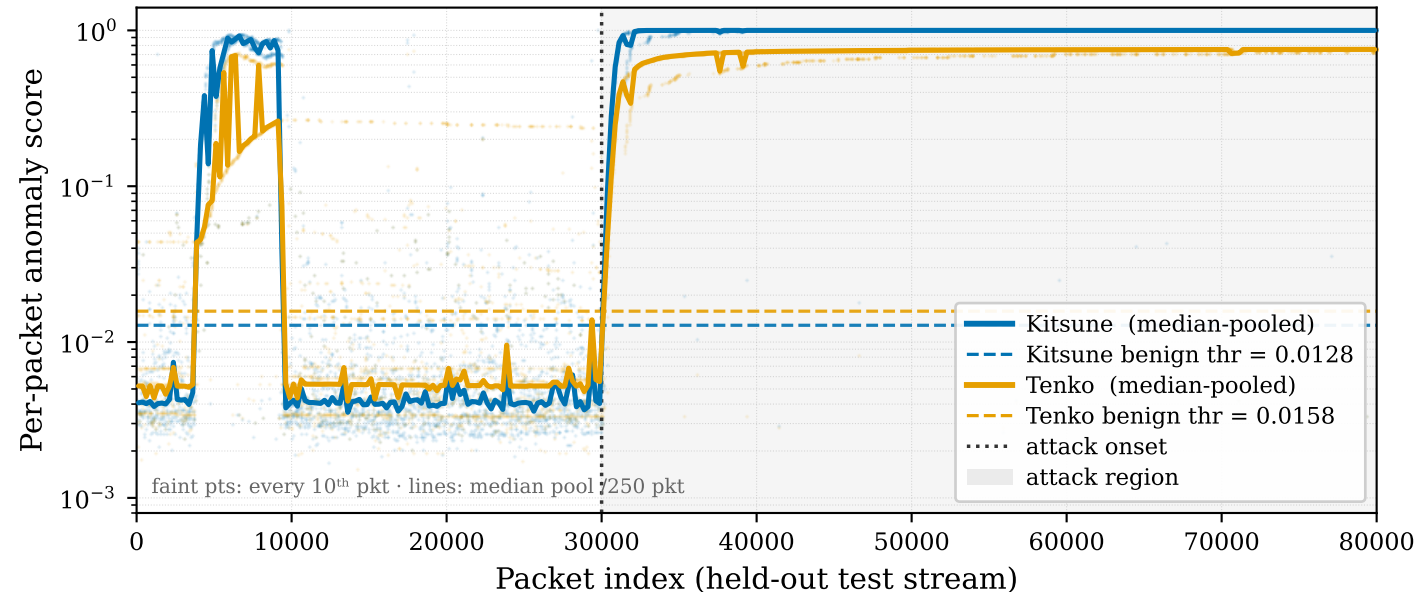
Tenko vs Kitsune anomaly score — DoS SYN Flood (CICIoT2023)
