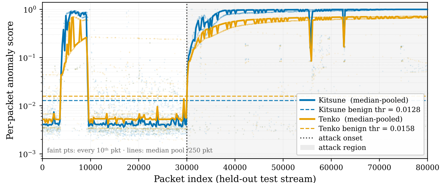
Tenko vs Kitsune anomaly score — MITM ARP Spoofing (CICIoT2023)
