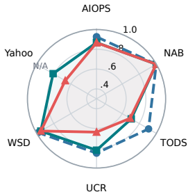
(b) Point-F1 (F1)
