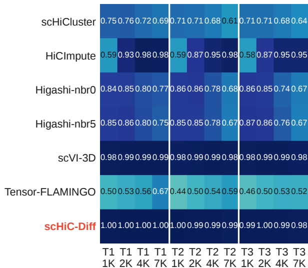
ROC-AUC
