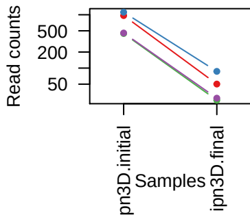
sgRNAs in PSMA5
