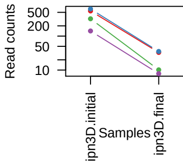
sgRNAs in PSMA5
