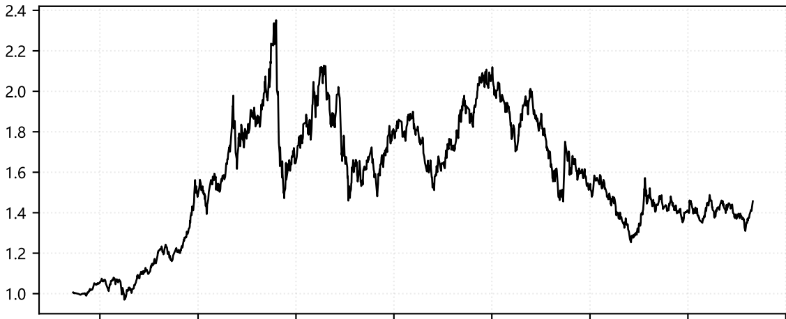
黑色系合成指数
