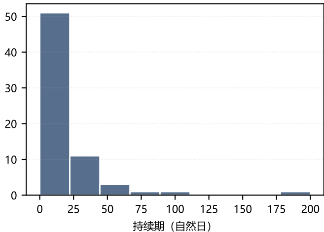
状态持续期分布 (均值 15 天)
