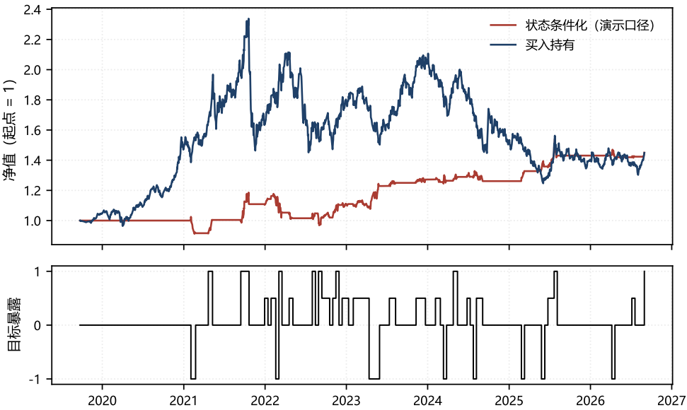
图 3: 条件化口径与买入持有的净值曲线（上）与目标暴露（下，阶梯线）
