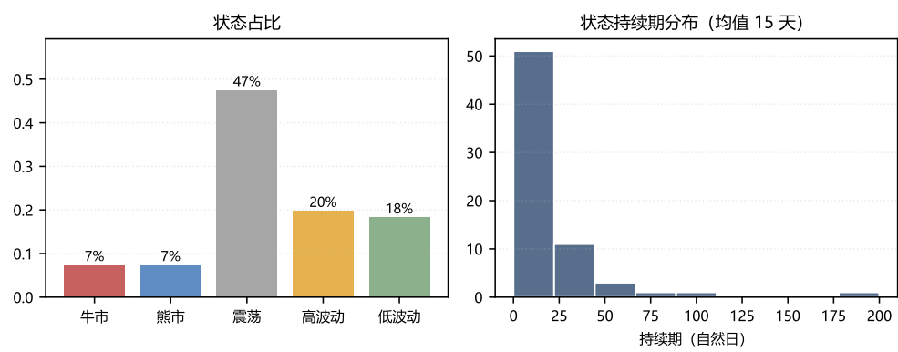
图 2: 各状态占比（左）与状态持续期分布（右）
