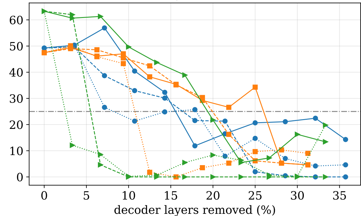
OBQA dataset
