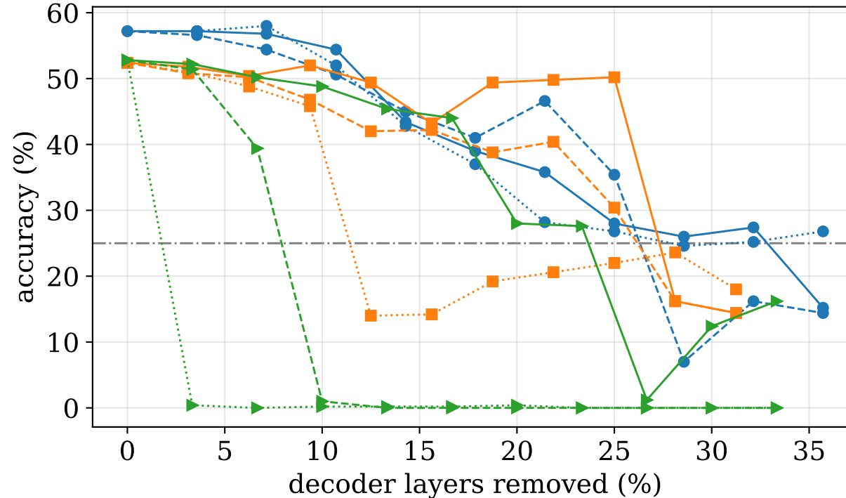
MMSU dataset
