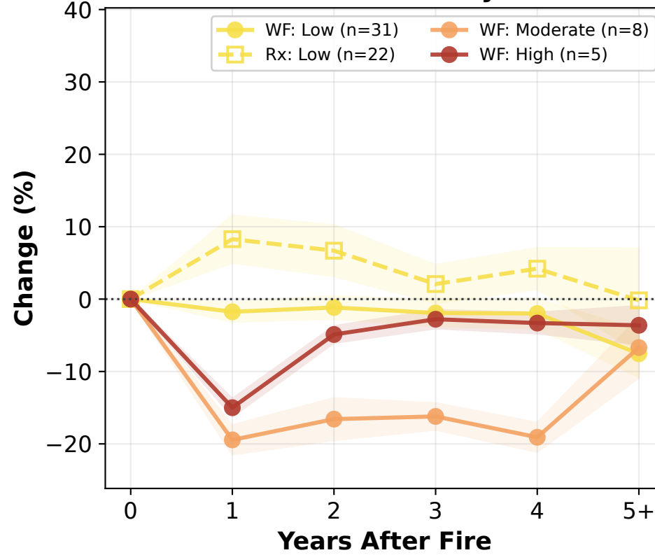
(B) Colorado: Fire Severity
