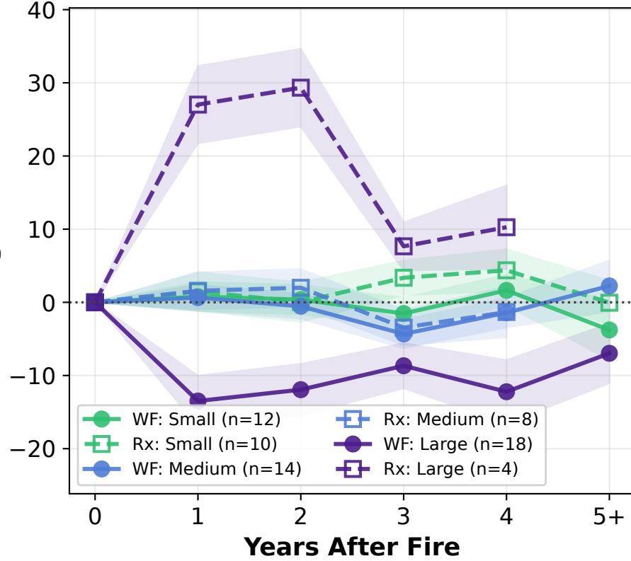
(A) Colorado: Fire Size
