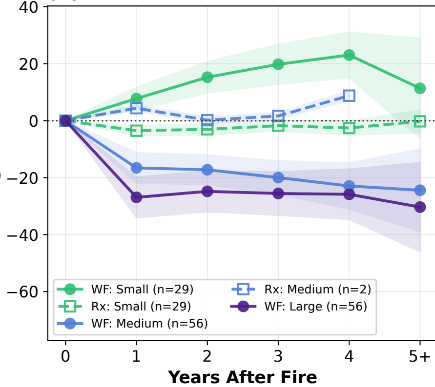
(D) California: Fire Size
