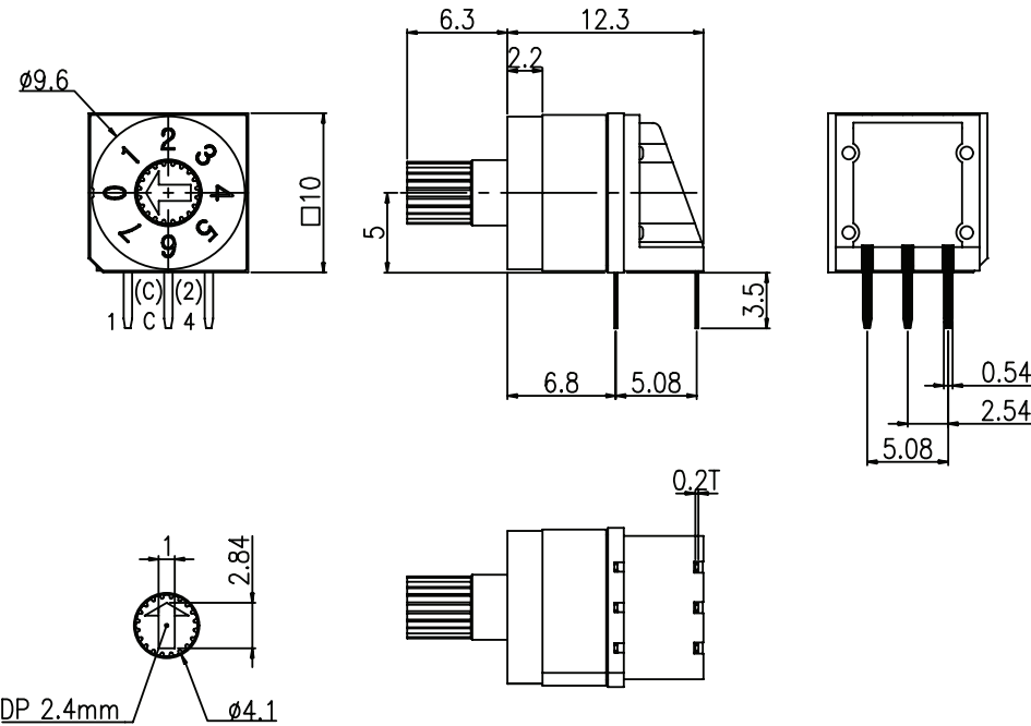
ACTUATOR
