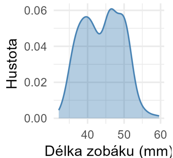
Graf hustoty
