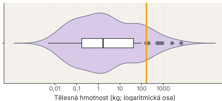
Obrázek 1: Oranžová svislá čára označuje aritmetický průměr, čára uvnitř krabice medián a šedé body možné odlehle hodnoty.
