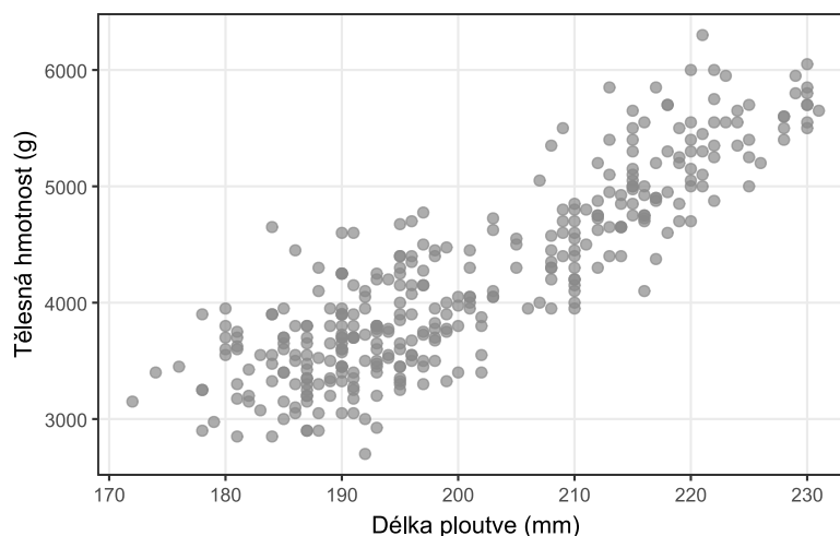
Obrázek 2: Bodový graf délky ploutve (mm) a tělesné hmotnosti (g) pro 333 tučňáků z datasetu Palmer Penguins.
