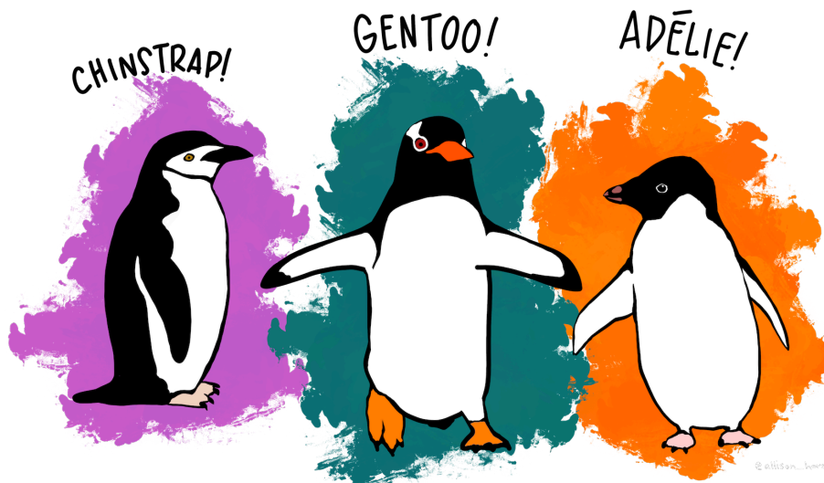
Obrázek 1: Tři druhy tučňáků v datasetu Palmer Penguins. Ilustrace: Allison Horst.
