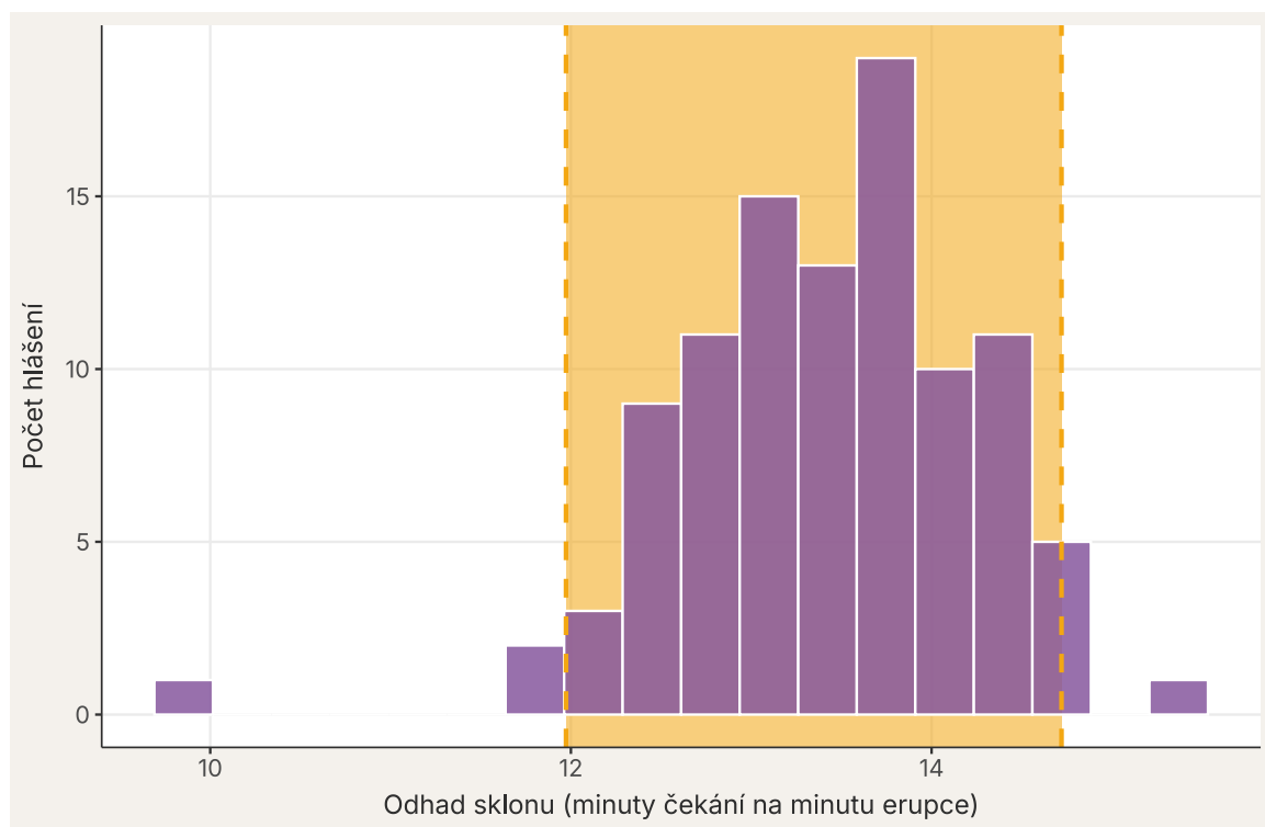
Obrázek 7: Kvantily rozdělují 100 sklonů z výukové demonstrace. Mezi svislými čarami leží prostředních 95 % jejich rozdělení.
