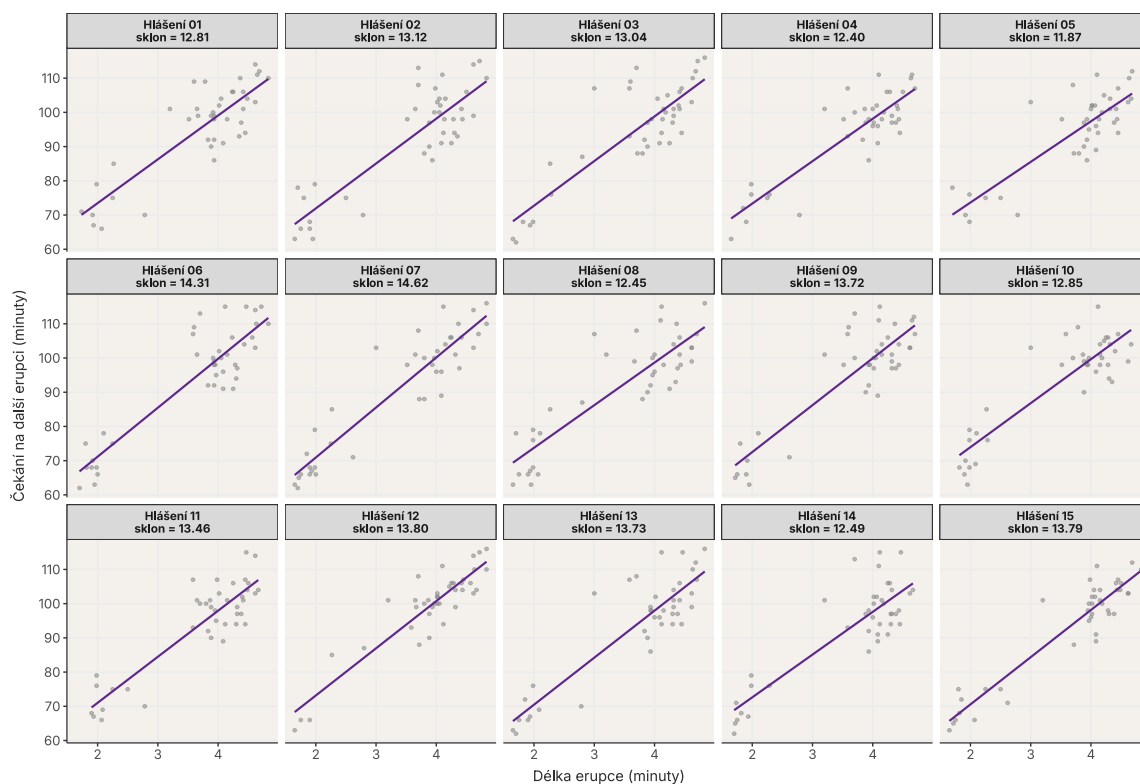
Obrázek 4: Patnáct náhodně vytvořených hlášení GeyserWatch. Každý panel obsahuje 40 erupcí, vlastní přímkou a vlastní sklon.
