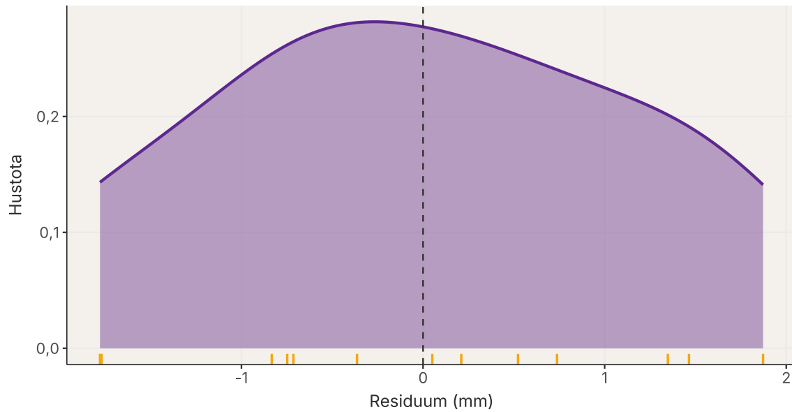
Obrázek 4: Vyhlazený odhad rozdělení residuí krabího modelu. Krátké čárky dole označují jednotlivé lokality.
