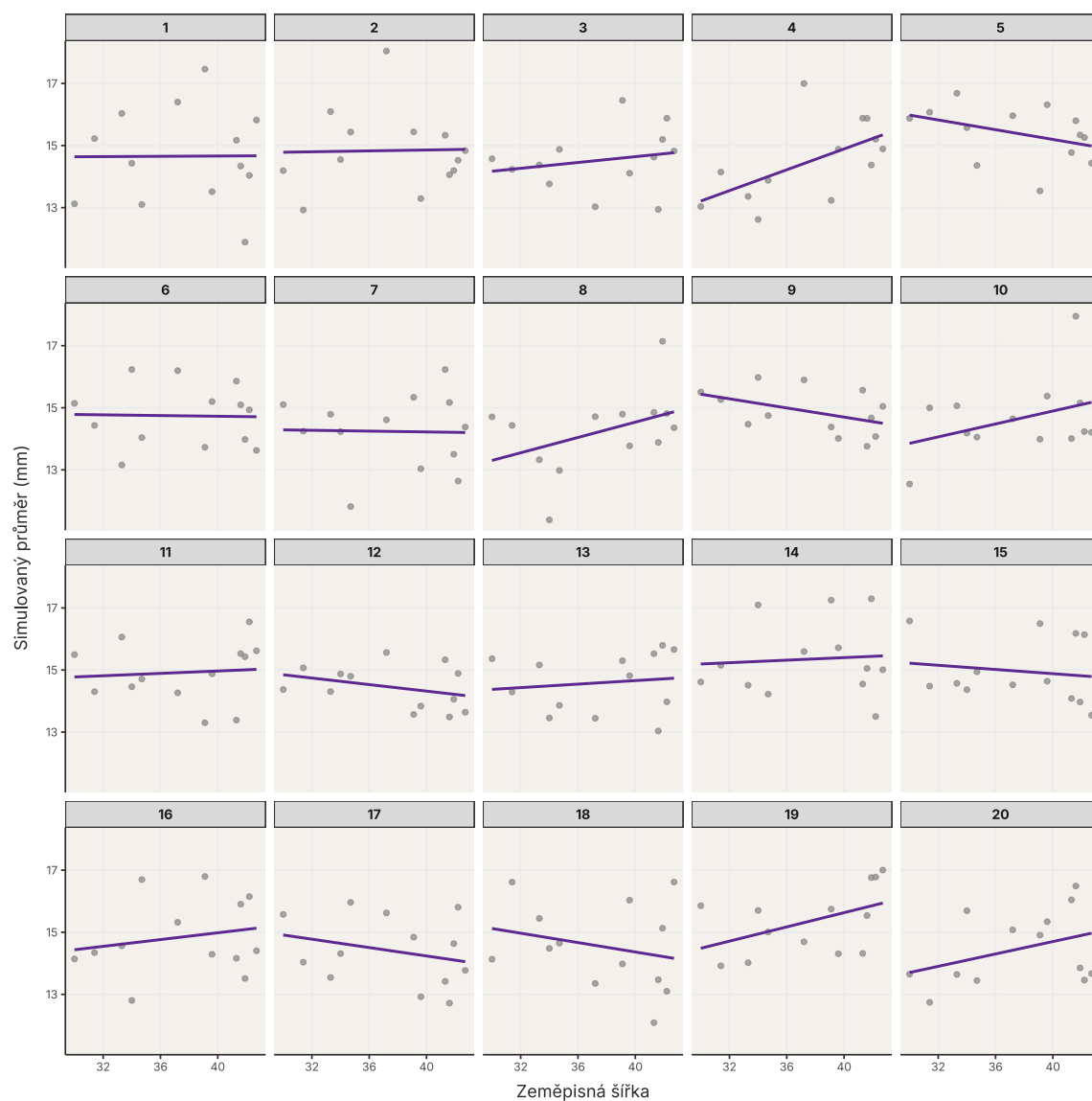
Obrázek 8: Dvacet náhodných studií vytvořených ve světě s nulovým sklonem. Od vodorovné přímky jsme ke každé lokalitě přičetli nové náhodné residuum. Každá studie obsahuje stejný počet bodů jako naše data a vlastní fitovanou přímku.
