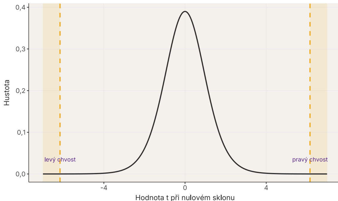
Obrázek 12: Oranžové pásy označují hodnoty t alespoň tak vzdálené od nuly jako pozorované t . Hledaný podíl tvoří plocha pod křivkou uvnitř obou pásů.
