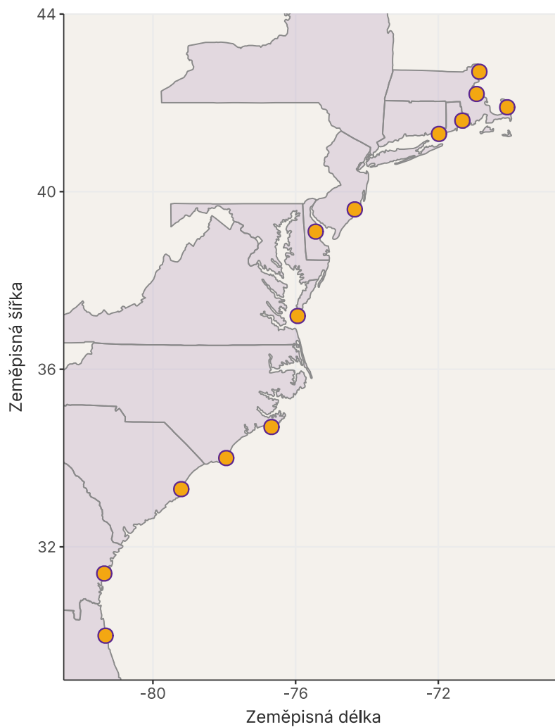
Obrázek 1: Každý oranžový bod představuje jedno sledované slanisko podél atlantského pobřeží USA. Souřadnice pocházejí z tabulky 1 související studie.
