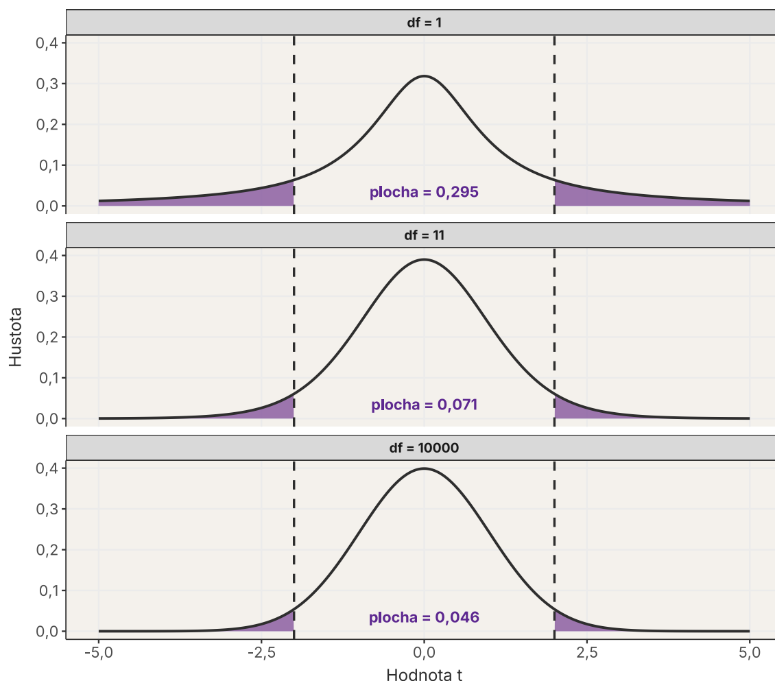
Obrázek 11: Ilustrační hranice t = -2 a t = 2 nejsou výsledkem krabího modelu. Ukazují pouze, že při menším df zůstává za stejnými hranicemi větší část celkové plochy.
