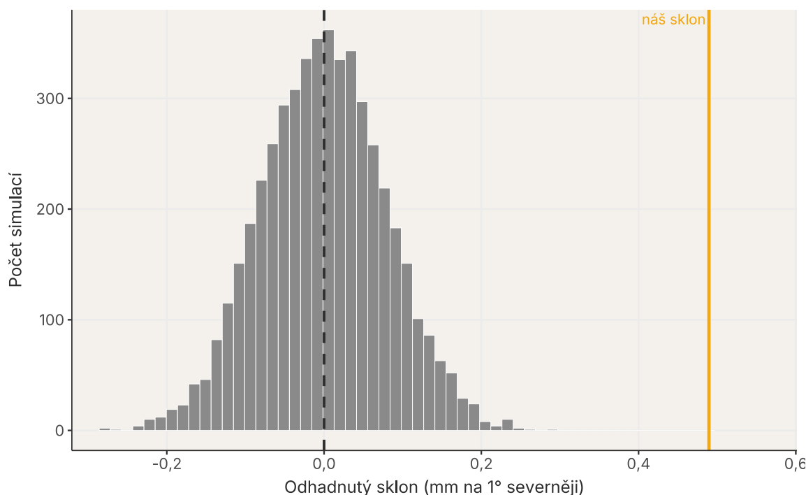
Obrázek 9: Sklony z 5 000 simulovaných souborů, ve kterých byl skutečný sklon nulový. Šedá čárkovaná čára označuje nulu, oranžová pozorovaný sklon.
