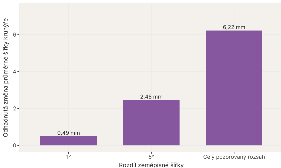
Obrázek 6: Tentýž sklon přepočtený na 1°, na zvolený větší rozdíl a na celý rozsah sledovaných zeměpisných šířek.
