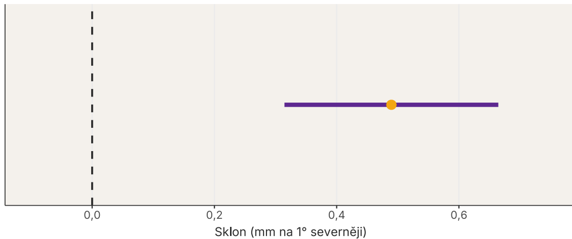
Obrázek 14: Odhad sklonu a jeho 95% interval spolehlivosti. Svislá čára označuje nulový sklon, tedy žádnou lineární změnu k severu.
