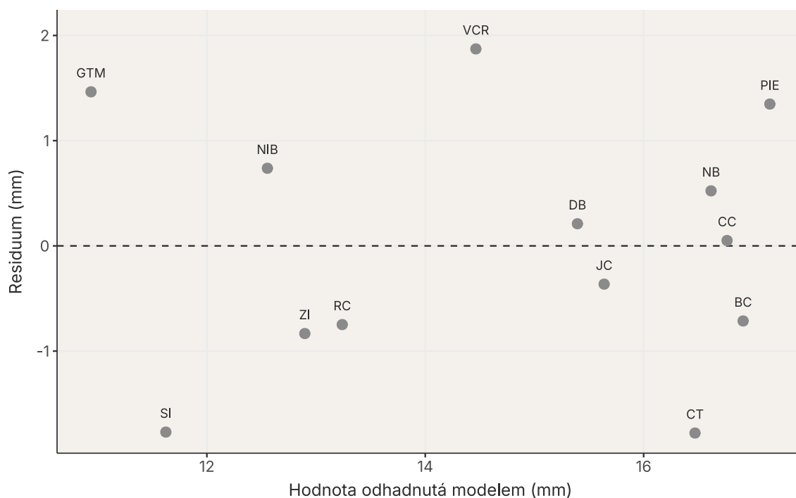
Obrázek 5: Residua proti hodnotám odhadnutým modelem. Popisky umožňují spojit neobvyklé residuum s konkrétní lokalitou.
