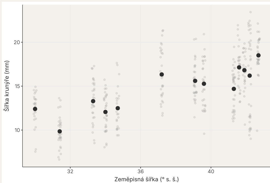
Obrázek 2: Jednotliví krabi sdílejí zeměpisnou šířku svého slaniska. Velké body zobrazují průměry použité v hlavním modelu.
