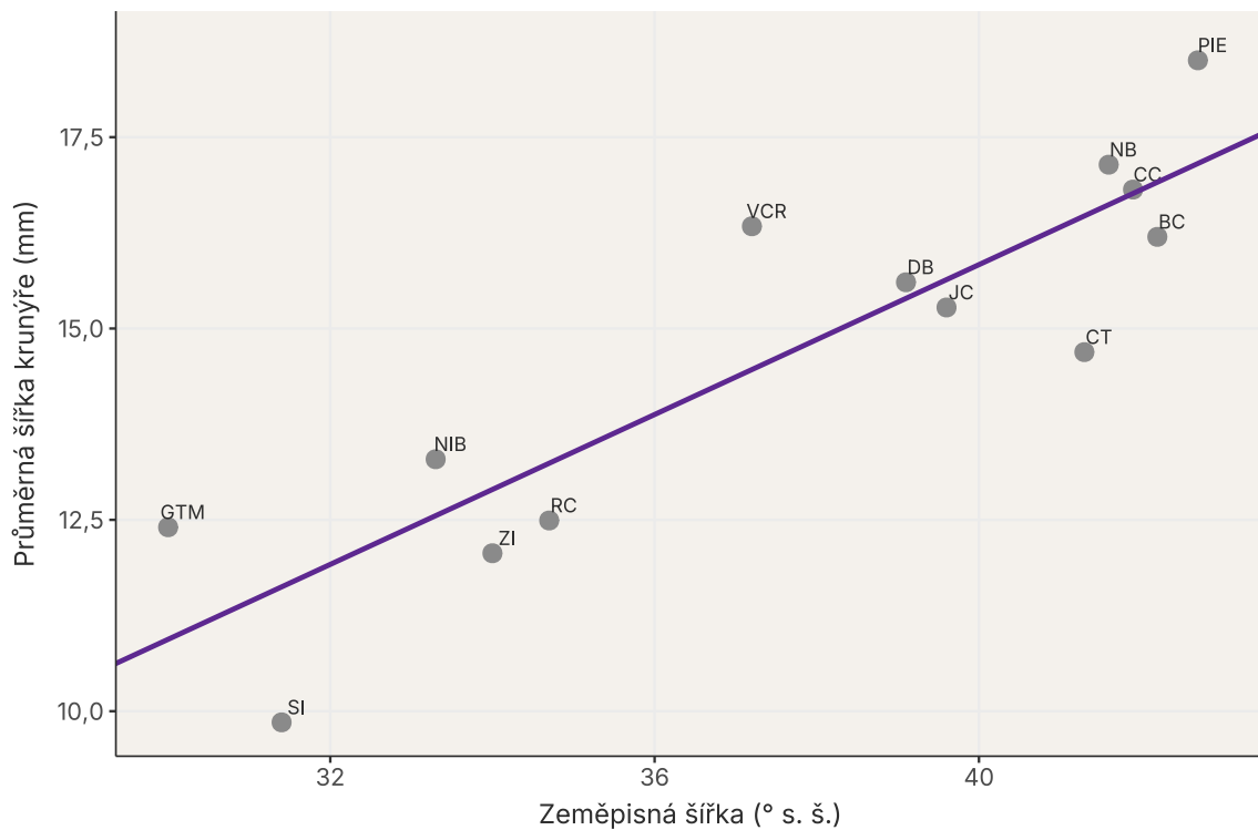
Obrázek 3: Průměrná šířka krunýře na sledovaných slaniskách. Fialová přímka je jednoduchý lineární model.
