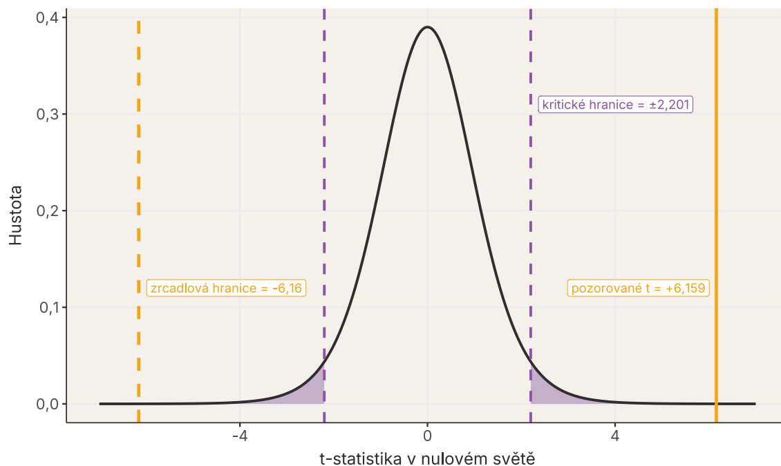
Obrázek 13: Kritické hranice a pozorovaná t-statistika v nulovém t-rozdělení. Fialové chvosty mají dohromady plochu alfa; oranžové hranice vymezují oboustrannou p-hodnotu.
