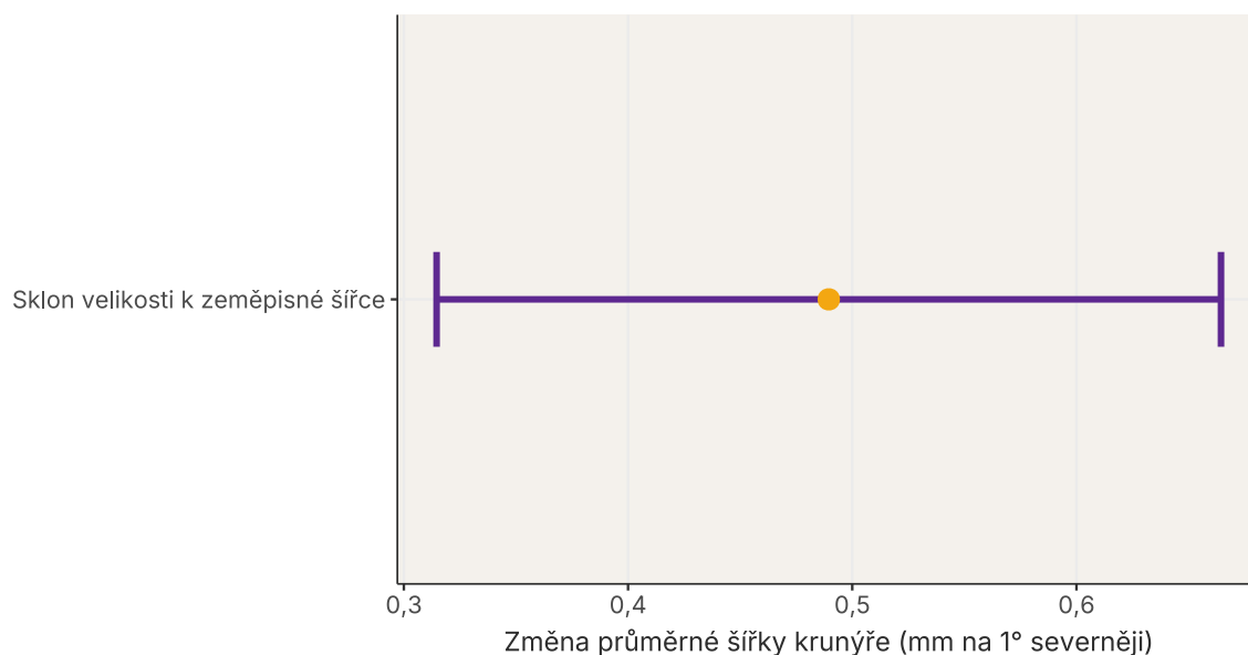
Obrázek 7: Odhad sklonu a jeho 95% interval spolehlivosti.
