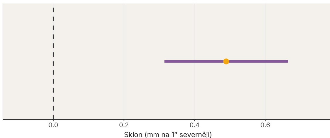
Obrázek 13: Odhad sklonu a jeho 95% interval spolehlivosti. Svislá čára označuje nulový sklon, tedy žádnou lineární změnu k severu.
