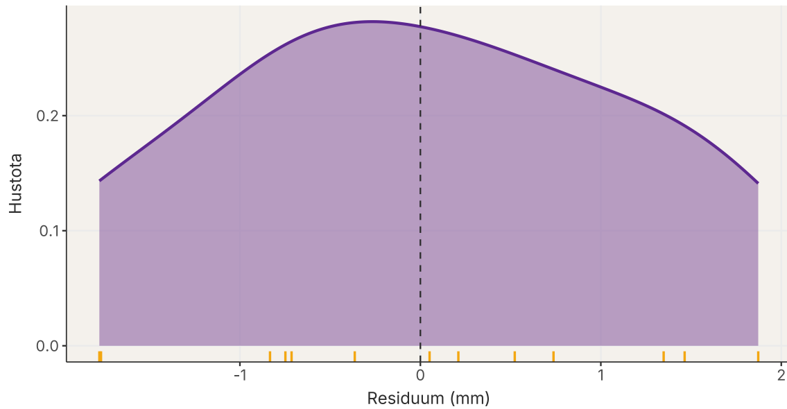
Obrázek 4: Vyhlazený odhad rozdělení třinácti residuí krabího modelu. Krátké čárky dole označují jednotlivé lokality.
