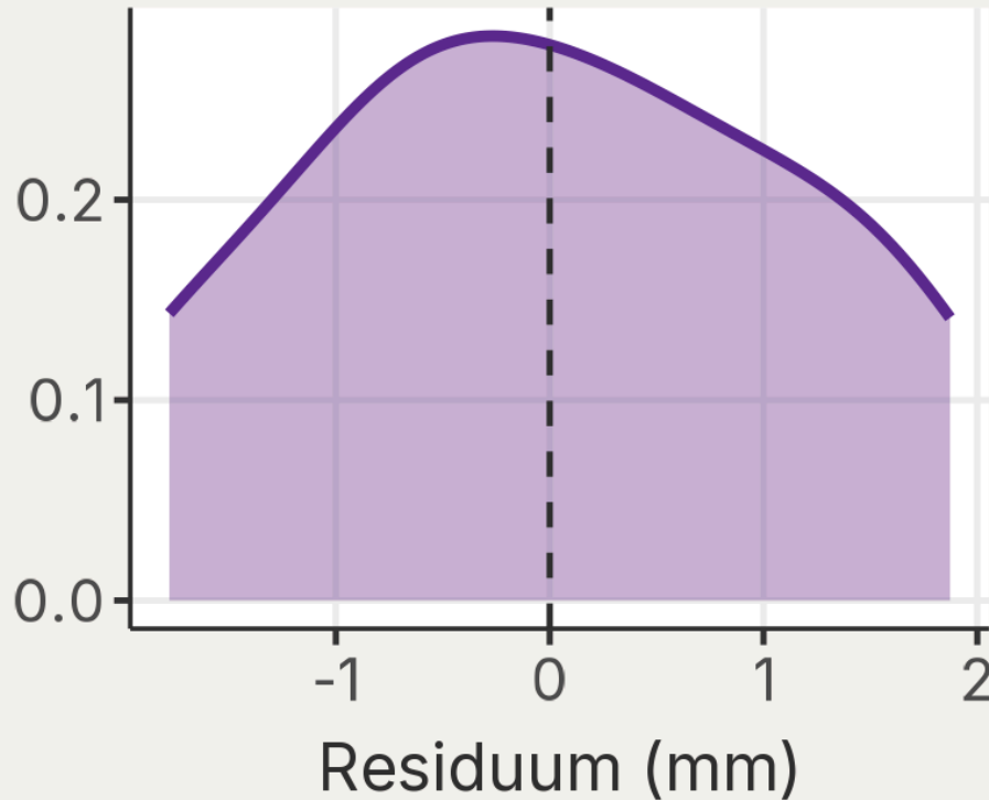
Rozdělení residuů
