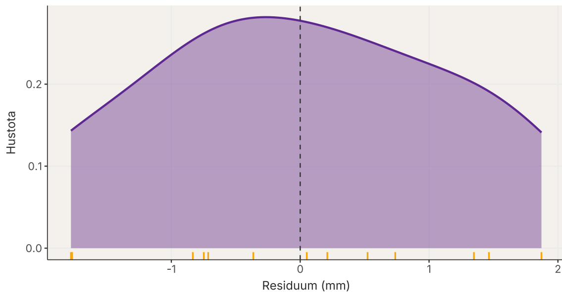
Obrázek 4: Vyhlazený odhad rozdělení třinácti residuů krabiho modelu. Krátké čárky dole označují jednotlivé lokality.
