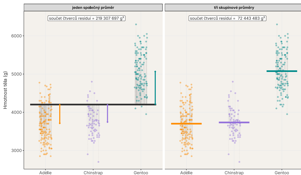
Obrázek 18: Stejná pozorování popsána jedním společným průměrem a třemi skupinovými průměry. Body jsou kvůli překryvu mírně posunuty do stran. Tečkované svislice jsou všechna residua; šipky v levém panelu ukazují posun od společného průměru k průměrům druhů.
