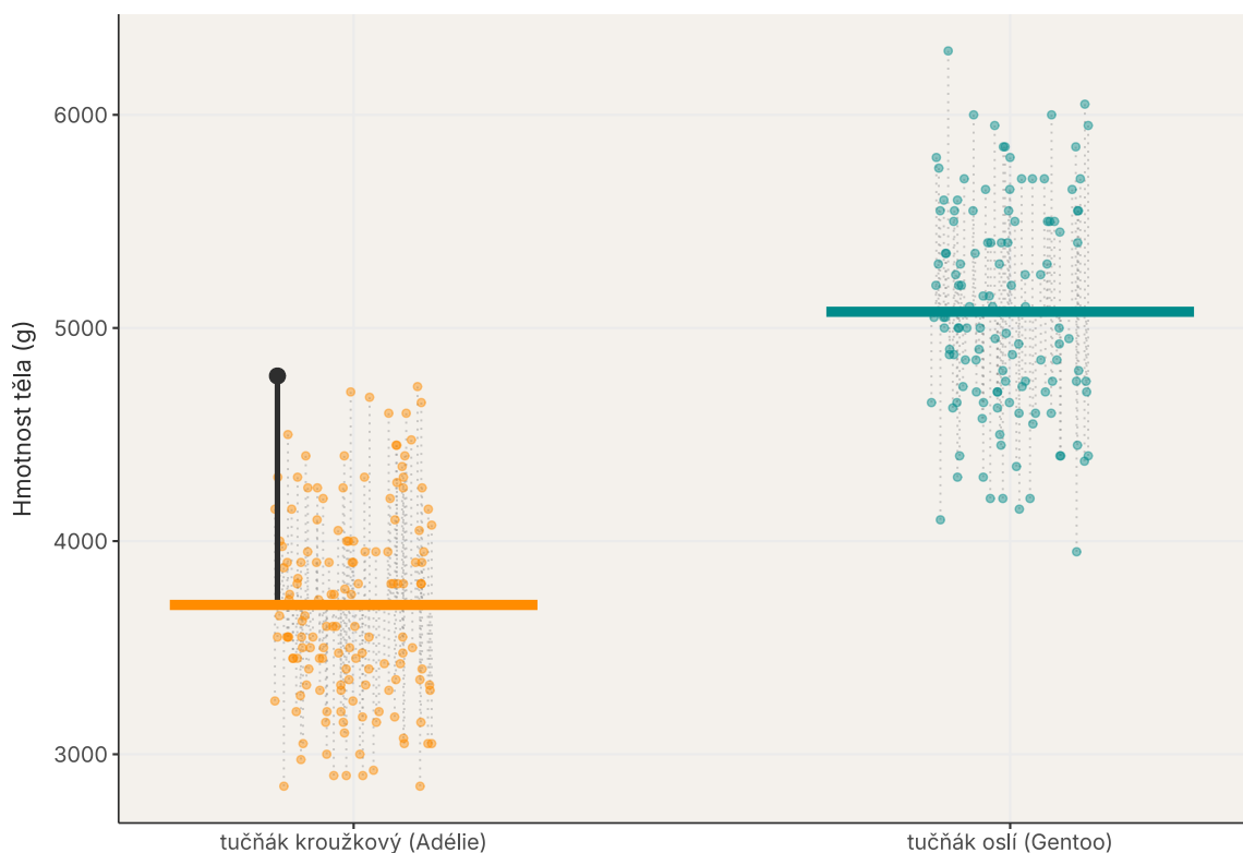
Obrázek 13: Každý jedinec sdílí odhadnutou hodnotu svého druhu. Body jsou kvůli překryvu mírně posunuty do stran. Tenké svislé úsečky spojují skutečné body s odhadem a jsou tedy residui; jedno residuum je zvýrazněno.
