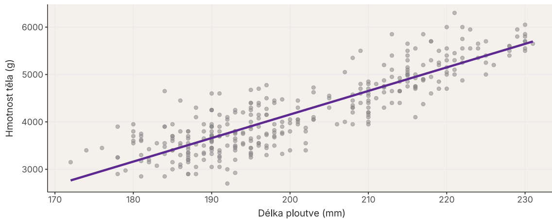
Obrázek 7: Pozorované délky ploutve a hmotnosti tučňáků s odhadnutou přímkou. Každá hodnota numerického prediktoru vybírá jedno místo na přímce.
