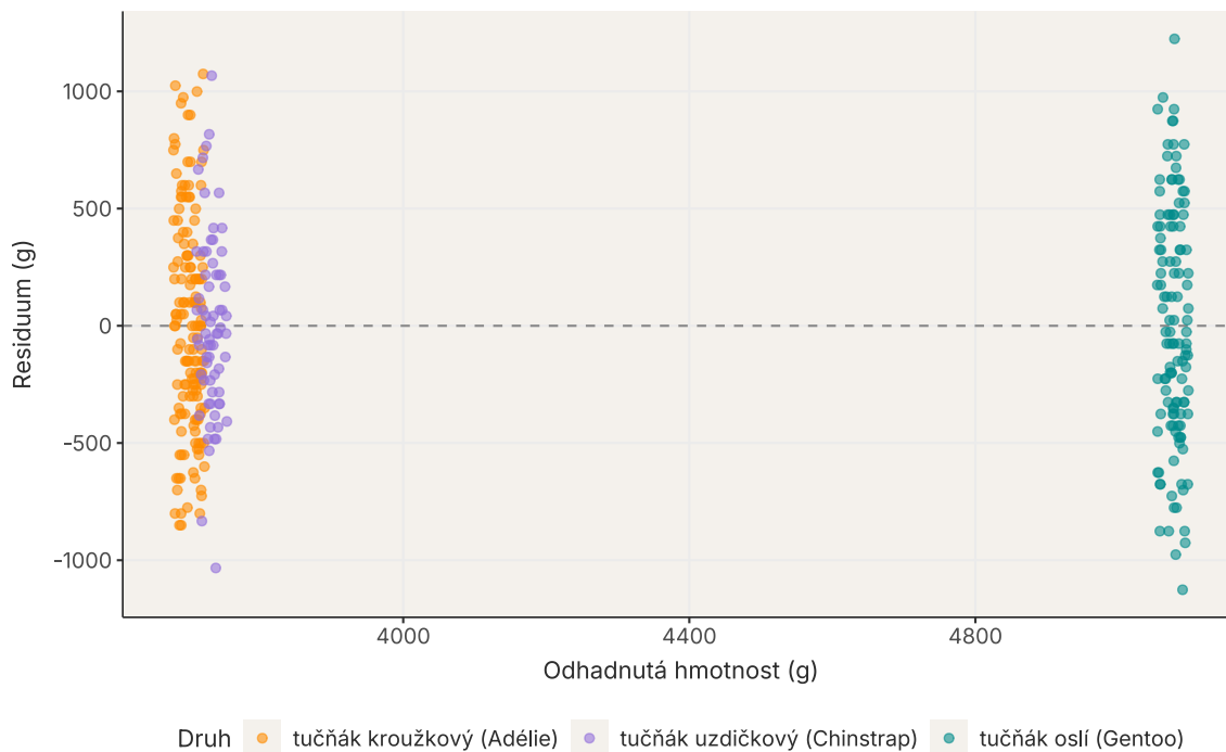
Obrázek 17: Residua proti odhadnutým hodnotám. Svislé pásy odpovídají skupinovým průměrům a jsou vlastností tohoto modelu, ne samy o sobě závadou. Pásy Adélie a Chinstrap téměř splývají, protože jejich průměry jsou skoro stejné.
