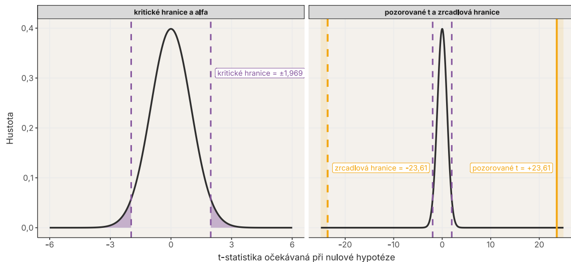
Obrázek 15: T-rozdělení při nulové hypotéze. Levý panel ukazuje kritické hranice a fialové chvosty o celkové ploše \alpha = 0,05 . V pravém panelu fialové čáry tyto hranice připomínají, zatímco oranžové pásy označují oblasti za pozorovaným t = 23,61 a zrcadlovou hranicí -23,61 . P-hodnota je plocha pod t-křivkou uvnitř těchto oranžových oblastí.
