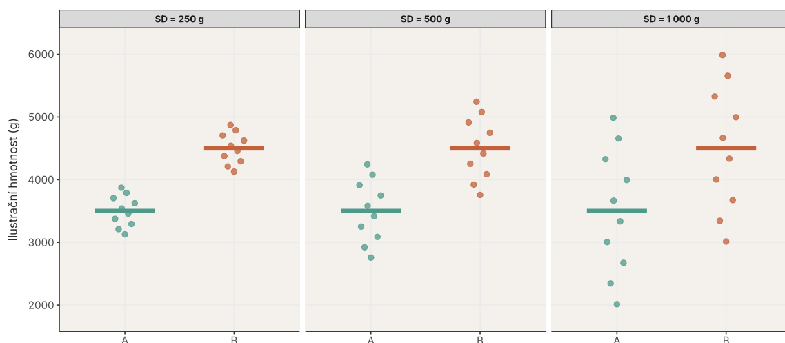
Obrázek 6: Myšlenkový pokus se dvěma vymyšlenými skupinami A a B: rozdíl mezi průměry (vodorovné úsečky) je ve všech třech panelech stejný, směrodatná odchylka uvnitř skupin zleva doprava roste.
