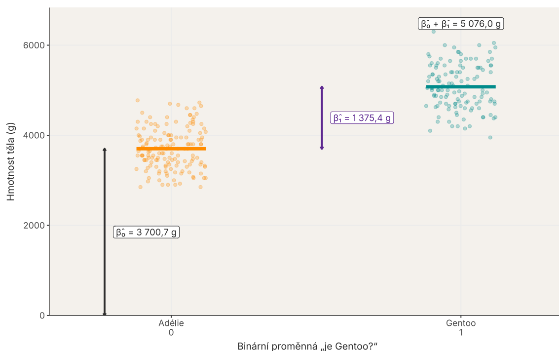
Obrázek 12: Dva koeficienty dvouskupinového modelu přímo v datech. Intercept \beta_0 je vzdálenost průměrové úsečky Adélie od nuly; koeficient \beta_1 je rozdíl Gentoo minus Adélie.
