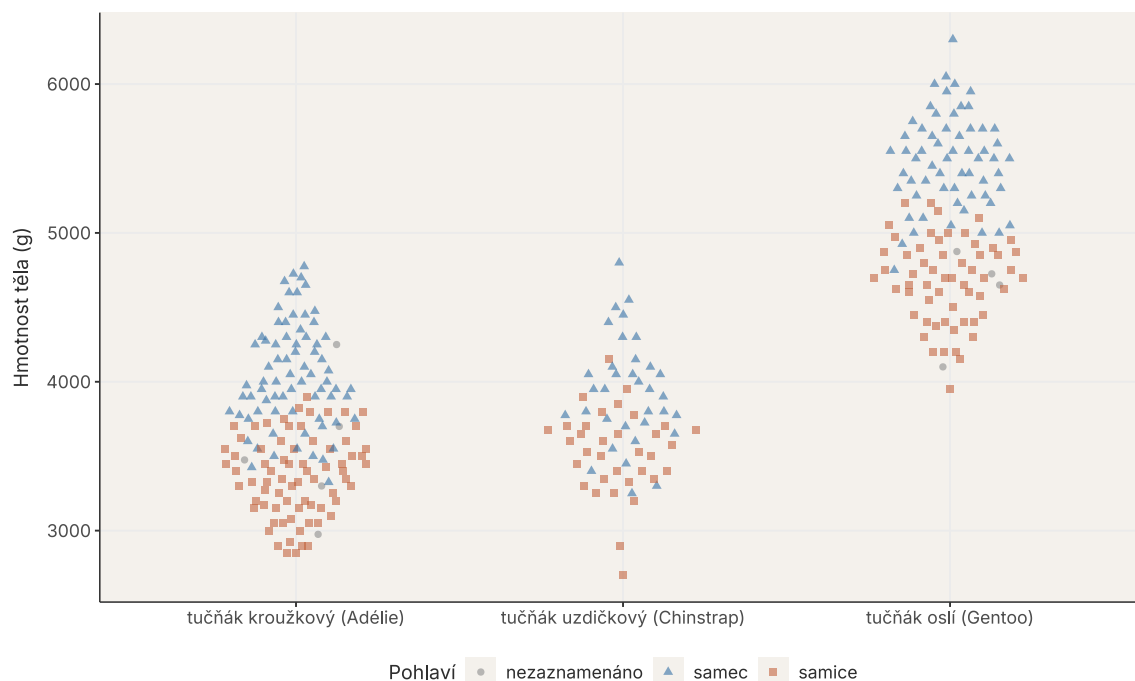
Obrázek 23: Hmotnosti tří druhů rozlišené podle zaznamenaného pohlaví. Šedé body mají pohlaví nezaznamenané.
