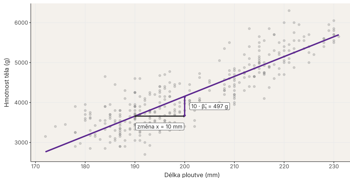
Obrázek 9: Sklon převádí změnu prediktoru na změnu odhadnuté hodnoty. Kvůli čitelnosti je zobrazena změna při prodloužení ploutve o 10 mm.
