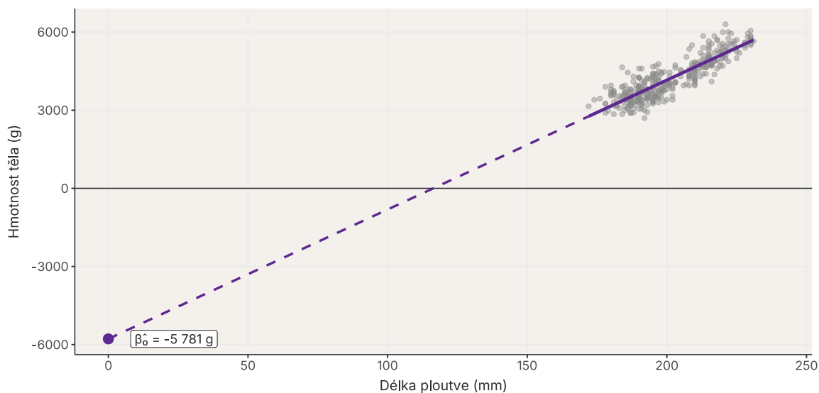
Obrázek 8: Intercept je výška přímky při hodnotě prediktoru 0. Čárkovaná část upozorňuje, že mezi nulou a nejkratší pozorovanou ploutví nemáme žádná data.
