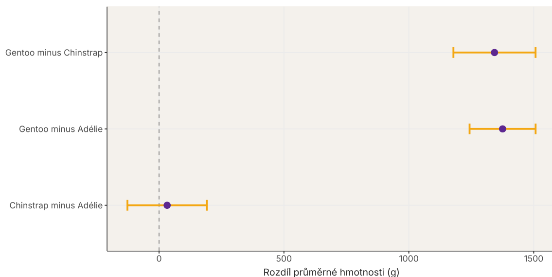
Obrázek 22: Tři Tukeyho post-hoc rozdíly a simultánní 95% intervaly. Nula znamená stejné průměry dané dvojice.
