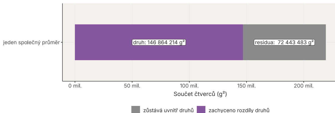
Obrázek 20: Původní součet čtverců residuí se po přidání druhu rozdělí na část zachycenou rozdíly skupinových průměrů a část, která stále zůstává uvnitř druhů.
