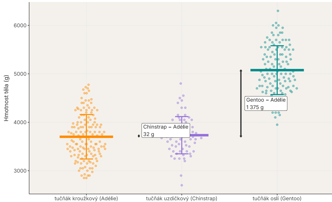
Obrázek 16: Tři druhy s průměrem \pm 1 SD. Svislé závorky ukazují oba rozdíly, které model přímo vyjadřuje vůči referenčnímu druhu Adélie.
