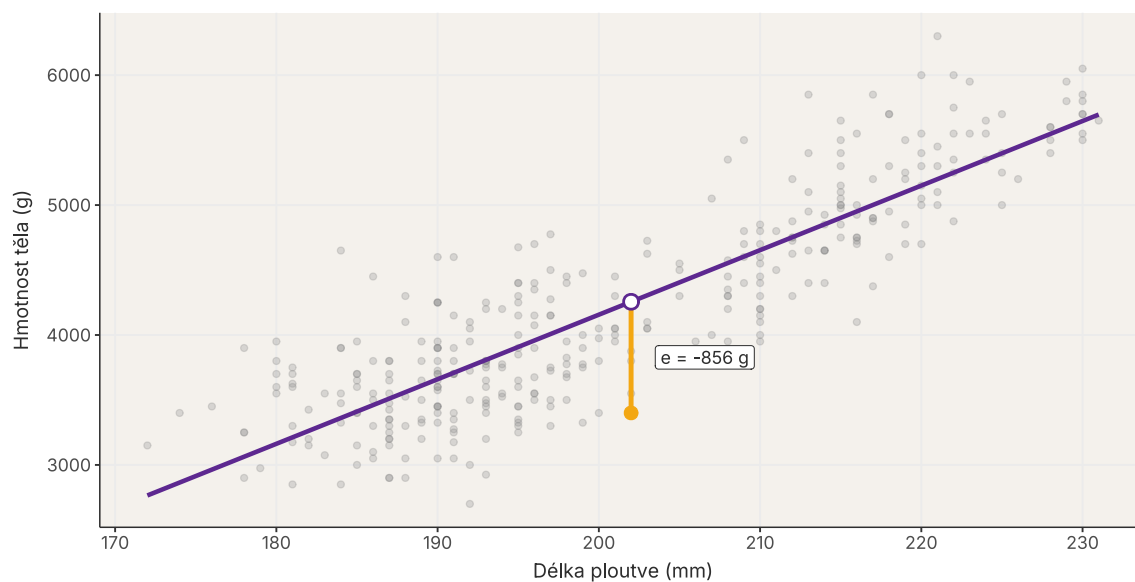
Obrázek 10: Residuum jednoho pozorování je svislá vzdálenost mezi naměřenou hodnotou (plný oranžový bod) a odhadnutou hodnotou na přímce (prázdný fialový bod).
