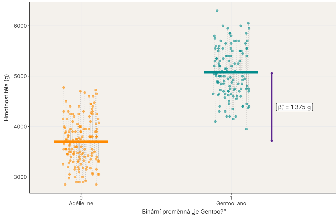
Obrázek 11: Kategorie druhu zapsaná binární proměnnou 0/1. Model přiřadí všem jedincům s hodnotou 0 průměr Adélie a všem jedincům s hodnotou 1 průměr Gentoo. Body jsou jen kvůli překryvu mírně posunuty do stran; tečkované úsečky jsou residua.
