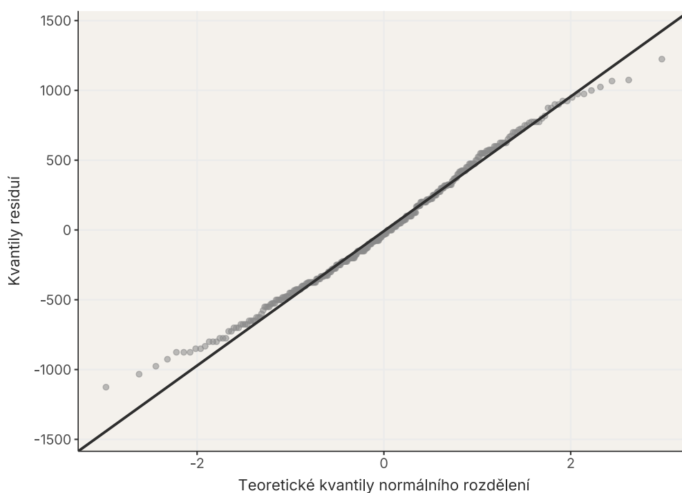
Obrázek 18: Q–Q graf residuí. Body převážně sledují referenční přímkou; menší odchylky na koncích jsou u reálných dat běžné.
