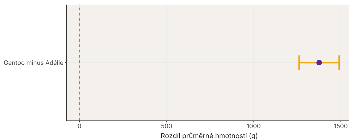
Obrázek 14: Odhad rozdílu průměrné hmotnosti Gentoo minus Adélie a jeho 95% interval spolehlivosti. Nula znamená stejné průměry.
