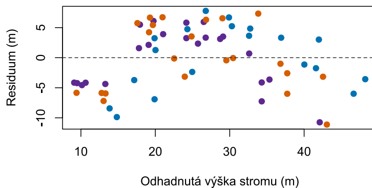
Obrázek 7: Residua aditivního modelu podle odhadnuté výšky.
