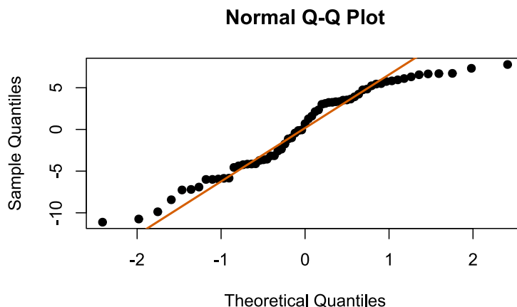
Obrázek 8: Q–Q graf residuí aditivního modelu.
