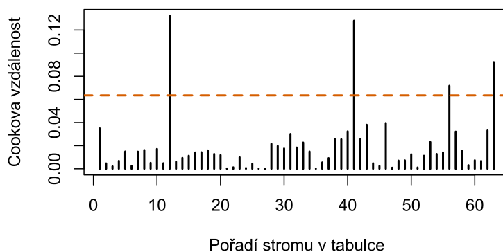
Obrázek 9: Cookovy vzdálenosti pro aditivní model. Přerušovaná čára zobrazuje orientační hodnotu 4/n .
