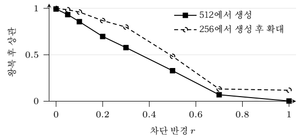
그림 7: 오토인코더에 넣은 조건과, 인코딩-디코딩 왕복 후 다시 추출한 조건 사이의 상관. FFHQ-512 파일 순서로 처음 24장이며 테스트 split이 아니다. r \approx 0.5 위에서는 조건이 사실상 사라진다. 조건을 256에서 만들어 확대하면 구조가 더 낮은 절대 주파수에 놓여 훨씬 많이 보존되며, 예전 파이프라인과 비교할 때 소스 해상도를 명시해야 하는 이유다.
