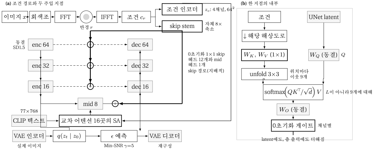
그림 2: (a) 반경 r 의 원판을 스펙트럼에서 제거하고, 학습되는 합성곱 인코더가 그 결과를 전체 해상도로 읽는다. VAE는 거치지 않는다. 그 특징은 동결 UNet에 두 번 들어간다. 디코더로 가는 각 skip 텐서에 0으로 초기화된 잔차로( \oplus ; 그림에는 해상도 세 단계와 mid block이 그려져 있고, 네트워크에는 skip 헤드 12개와 mid 헤드 하나가 있다), 그리고 교차 어텐션 16곳의 StandAlone 어텐션으로. 선 굵기는 측정된 분배를 따른다. r=0 에서 skip 경로만 켜면 SC가 0.5370, 어텐션만 켜면 0.2112다(5.2절). (b) StandAlone 한 지점. 쿼리는 UNet 자신의 latent에서 동결 W_Q 를 거쳐 오고, 키와 값은 조건에서 학습된 1×1 투영을 거쳐 온다. unfold로 각 위치가 전체 맵이 아니라 자기 3×3 이웃만 참조한다. 1×1 창도 적어도 그만큼 잘 작동한다(5.2절). 결과는 동결 출력 투영과 0초기화 채널별 게이트를 지나, latent에 더해져 아래의 텍스트 쿼리가 구조를 보게 하고, 층이 반환하는 값에도 더해진다.
