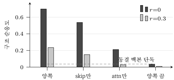
그림 6: 두 주입 경로를 모두 켜 경우, 각각 단독, 그리고 둘 다 끈 경우. skip 잔차가 구조 신호의 대부분을 나르고, 교차 어텐션 단독으로는 거의 회복하지 못하며, 둘 다 끄면 동결 백본으로 떨어진다(FID 120.50, 양쪽 켜는 때는 50.13). 두 경로는 거의 가산적이다.
