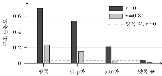
그림 8: 두 주입 경로를 모두 켜 경우, 각각 단독, 그리고 둘 다 끈 경우. skip 잔차가 구조 신호의 대부분을 나르고, 교차 어텐션 단독으로는 거의 회복하지 못하며, 둘 다 끄면 동결 백본으로 떨어진다(FID 120.50, 양쪽 켜올 때는 50.13, skip만 65.12, 어텐션만 67.07). 점선은 r=0 에서 양쪽을 끈 대조군이다. r=0 에서는 대조군 대비 단일 경로 이득의 합이 양쪽 경로 점수와 대략 같고, r=0.3 에서는 양쪽 경로가 그 합을 넘는다.
