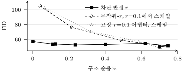
그림 4: 위: 차단 반경이 커질수록 구조 순응도는 내려가고 표본 다양성은 올라간다. 아래: 표 1의 차단 반경 스윙과 표 2의 두 스케일 어댑터를 구조 순응도/FID 평면에 놓은 것. 조건의 대역폭을 좁히면 좁은 FID 대역 안에서 구조 순응도가 내려가고, 어느 어댑터든 약하게 하면 FID가 오르며 내려간다. 스케일한 점은 r_m=0.1 로, 차단 반경 점은 각자의 차단 반경으로 채점했다. 두 패널 모두 평가출력에서 직접 그렸다.
