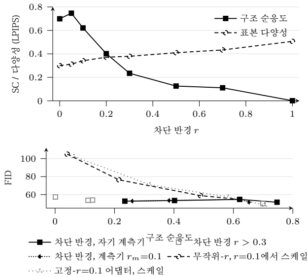
그림 4: 위: 차단 반경에 대한 구조 순응도와 표본 다양성(표 1의 값이며 SEM과 시드 sd도 거기에 있다). 아래: 구조 순응도에 대한 FID, 점마다 FID 추정은 하나다. 채운 사각형은 r \in [0.05, 0.3] 에서 자기 차단 반경으로 채점한 스윕, 빈 회색 사각형은 같은 스윕의 구간 밖이다. 마름모는 같은 생성물을 제측기 r_m=0.1 로 다시 채점한 것이다. 원과 삼각형은 무작위-r 어댑터와 고정-r=0.1 어댑터를 r=0.1 에서 스케일한 것으로, 이미 r_m=0.1 을 쓴다. 그 한 제측기에서 차단 반경 r=0.3 은 FID 52.77에서 0.2599에, 세기 0.50은 FID 76.46에서 0.2146에 이른다. 두 패널 모두 평가 출력에서 직접 그렸다.
