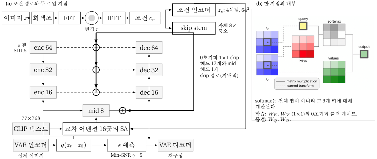
그림 2: (a) 반경 r 의 원판을 스펙트럼에서 제거하고, 학습되는 합성곱 인코더가 그 결과를 전체 해상도로 읽는다. VAE는 거치지 않는다. 그 특징은 동결 UNet에 두 번 들어간다. 디코더로 가는 각 skip 텐서에 0으로 초기화된 잔차로( \oplus ; 그림에는 해상도 세 단계와 mid block이 그려져 있고, 네트워크에는 skip 헤드 12개와 mid 헤드 하나가 있다), 그리고 교차 어텐션 16곳의 StandAlone 어텐션으로. 선 굵기는 측정된 분배를 따른다. r=0 에서 skip 경로만 켜면 SC가 0.5370, 어텐션만 켜면 0.2112다(5.2절). (b) StandAlone 한 지점. 쿼리는 UNet 자신의 latent에서 동결 W_Q 를 거쳐 오고, 키와 값은 조건에서 학습된 1 \times 1 투영을 거쳐 온다. unfold로 각 위치가 전체 맵이 아니라 자기 3 \times 3 이웃만 참조한다. 1 \times 1 창도 적어도 그만큼 잘 작동한다(5.2절). 결과는 동결 출력 투영과 0초기화 채널별 게이트를 지나, latent에 더해져 아래의 텍스트 쿼리가 구조를 보게 하고, 층이 반환하는 값에도 더해진다.
