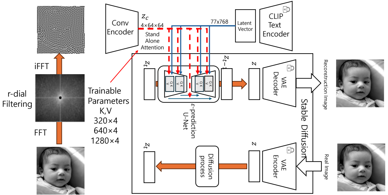
그림 2: 반경 r 의 원판을 스펙트럼에서 제거하고, 학습되는 합성곱 인코더가 그 결과를 전체 해상도로 읽어 VAE를 거치지 않고 4채널 64×64의 조건 z_c 를 만든다. 이는 동결 UNet의 교차 어텐션 16곳으로 들어가며, 그곳에서 학습되는 것은 W_K , W_V 와 0초기화 출력 게이트뿐이고 W_Q 와 W_O 는 동결이다(그림 3). 같은 조건 경로의 일부로 그려진 두 번째 학습 stem은 원본 조건을 읽어 디코더 skip 텐서 12곳과 mid block에 0초기화 잔차를 더한다. 구조의 대부분은 그 경로가 나르며, 분배는 측정된 값이다. r=0 에서 skip 경로만 켜면 SC가 0.5370, 어텐션만 켜면 0.2112다(5.2절). 학습은 Min-SNR 가중의 \epsilon 예측이고, 동결 오토인코더를 지나는 루프는 표준 잡재 확산 그대로이며 학습되지 않는다.
