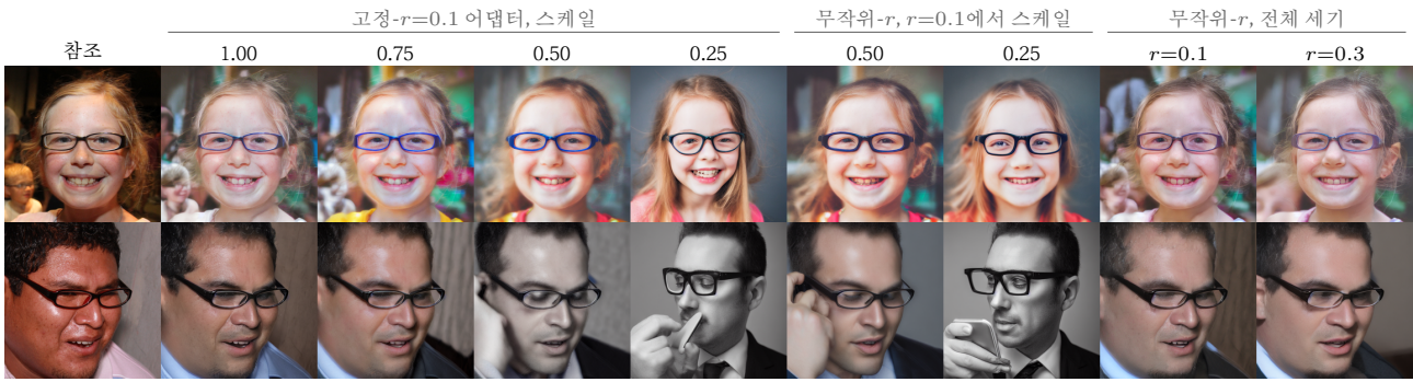
그림 6: 처음 두 테스트 이미지에 대한 어댑터 세기와 차단 반경. 샘플링 시드 2026과 BLIP 캡션을 전체에 걸쳐 고정했다. 2-5열은 고정- r=0.1 특화 모델을 세기 1.00에서 0.25까지 스케일한 것이다(표 2). 6-7열은 무작위- r 어댑터를 r=0.1 에서 0.50과 0.25로 스케일한 것이다. 8-9열은 같은 어댑터를 전체 세기로 r=0.1 (표 1)과 r=0.3 에서 돌린 것으로, 그림 4과 같은 생성물이다. 세기 0.75의 고정- r 어댑터는 여전히 참조를 따른다. 어느 어댑터든 세기를 0.50으로 낮추면 배경과 색이 바뀌고 둘째 행은 자세도 바뀐다. 0.25에서는 두 행 모두 자세와 구도가 바뀌고 둘째 행은 회색조가 된다. 차단 반경을 r=0.3 으로 옮기면 참조의 배치가 유지된다. 모든 출력은 이 논문이 다루는 모델이 생성한 것이다.
