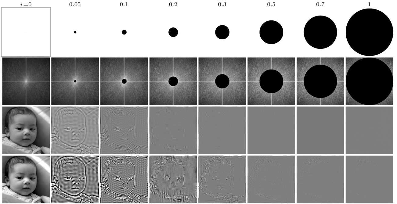
그림 1: 주과수 쪽에서 본 다이얼. 열은 r = 0, 0.05, 0.1, 0.2, 0.3, 0.5, 0.7, 1.0 이다. 1행: 방사형 마스크, 검은 부분이 제거된다. 2행: 마스크링 후 로그 크기 스펙트럼으로, 구멍이 바깥으로 커진다. 3행: 모델이 실제로 받는 조건. 4행: 같은 데이터를 \pm 2\sigma 로 표시해 남아 있는 내용을 드러낸 것. r \approx 0.2 위에서 조건은 평평한 회색으로 보이고 테스트 이미지 500장 평균 표준편차도 r=0 의 0.238에서 r=1 의 0.034로 떨어지지만, 4행에는 얼굴 윤곽이 남아 있고 모델은 r=0.2 에서 SC 0.4019에 도달한다. 이미지별 정규화 때문에 모델이 구조를 읽을 수 있는 것은 이 낮은 대비의 잔여뿐이다.
