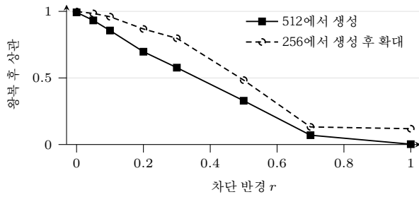
그림 8: 오토인코더에 넣은 조건과, 인코딩-디코딩 왕복 후 다시 추출한 조건 사이의 상관. FFHQ-512 파일 순서로 처음 24장이며 테스트 split이 아니다. r \approx 0.5 위에서는 조건이 사실상 사라진다. 조건을 256에서 만들어 확대하면 구조가 더 낮은 절대 주파수에 놓여 훨씬 많이 보존되며, 예전 파이프라인과 비교할 때 소스 해상도를 명시해야 하는 이유다.
