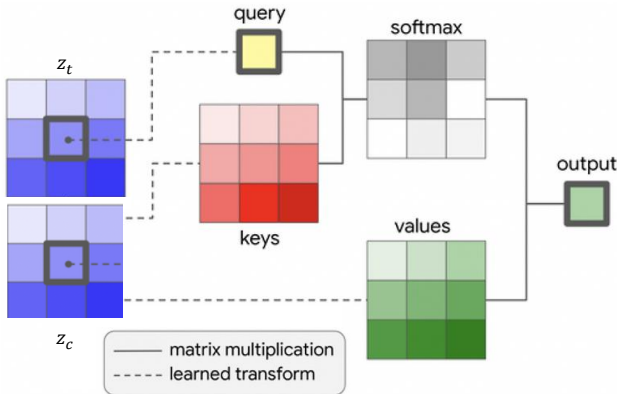
그림 3: StandAlone 한 지점. 쿼리는 UNet latent z_t 의 한 위치이고, 키와 값은 조건 z_c 에서 같은 위치의 3×3 이웃이다. 따라서 softmax는 전체 맵이 아니라 9개에 대해 계산되며, 1×1 창도 적어도 그만큼 잘 작동한다(5.2절). W_K , W_V 와 0초기화 채널별 게이트가 학습되고 W_Q 와 출력 투영은 동결이다. 게이트를 지난 결과는 latent에 더해져 아래의 텍스트 쿼리가 구조를 보게 하고, 층이 반환하는 값에도 더해진다.
