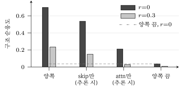
그림 9: 두 주입 경로를 모두 켜 경우, 각각 단독, 그리고 둘 다 끈 경우. skip 잔차가 구조 신호의 대부분을 나르고, 교차 어텐션 단독으로는 거의 회복하지 못하며, 둘 다 끄면 동결 백본으로 떨어진다(FID 120.50, 양쪽 켜올 때는 50.13, skip만 65.12, 어텐션만 67.07). 점선은 r=0 에서 양쪽을 끈 대조군이다. 경로는 학습된 주 모델에서 추론 시에 끈 것이며, 따로 학습한 skip 단독 모델은 표 6에 있다. r=0 에서는 대조군 대비 단일 경로 이득의 합이 양쪽 경로 이득과 대략 같고, r=0.3 에서는 양쪽 경로의 이득이 단일 경로 이득의 합을 넘는다.
