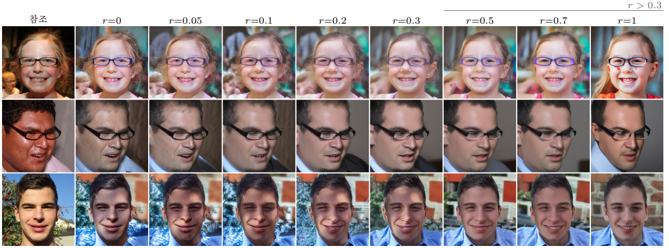
그림 4: 주 모델(학습 시드 2026)을 샘플링 시드 2026과 각 참조의 BLIP 캡션으로 돌린 것이며, 한 행 안에서는 r 만 바뀐다. 행은 테스트 이미지의 처음 세 장을 생성 순서대로 실은 것이고, 타일은 표 1에서 채점된 바로 그 저장된 생성물이다. 참조 이미지는 모델에 주어지지 않는다. r 이 커질수록 배경의 세부가 열어지고 옷과 색이 참조에서 멀어지지만 얼굴 배치는 유지되며, r=1 에서는 첫 행에 색 인공물이 나타난다. 모든 출력은 이 논문이 다루는 모델이 생성한 것이다.
