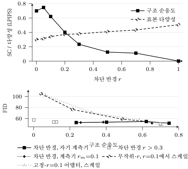
그림 5: 위: 차단 반경에 대한 구조 순응도와 표본 다양성(표 1의 값이며 SEM과 시드 sd도 거기에 있다). 아래: 구조 순응도에 대한 FID, 점마다 FID 추정은 하나다. 채운 사각형은 r \in [0.05, 0.3] 에서 자기 차단 반경으로 채점한 스윕, 빈 회색 사각형은 같은 스윕의 구간 밖이다. 마름모는 같은 생성물을 제측기 r_m=0.1 로 다시 채점한 것이다. 원과 삼각형은 무작위-r 어댑터와 고정-r=0.1 어댑터를 r=0.1 에서 스케일한 것으로, 이미 r_m=0.1 을 쓴다. 그 한 제측기에서 차단 반경 r=0.3 은 FID 52.77에서 0.2599에, 세기 0.50은 FID 76.46에서 0.2146에 이른다. 두 패널 모두 평가 출력에서 직접 그렸다.
