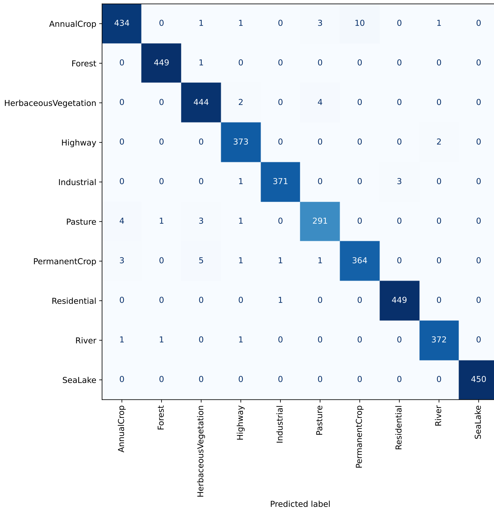
True label
