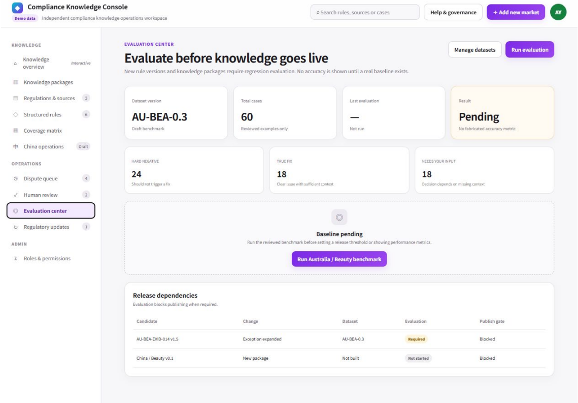
图 7 演示评测中心：未运行真实基准前不展示虚构准确率，发布状态保持 Blocked。
