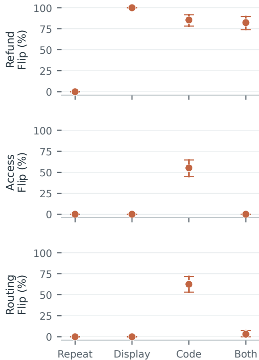
Llama 8B
