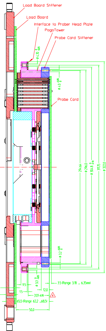
SECTION A-A
