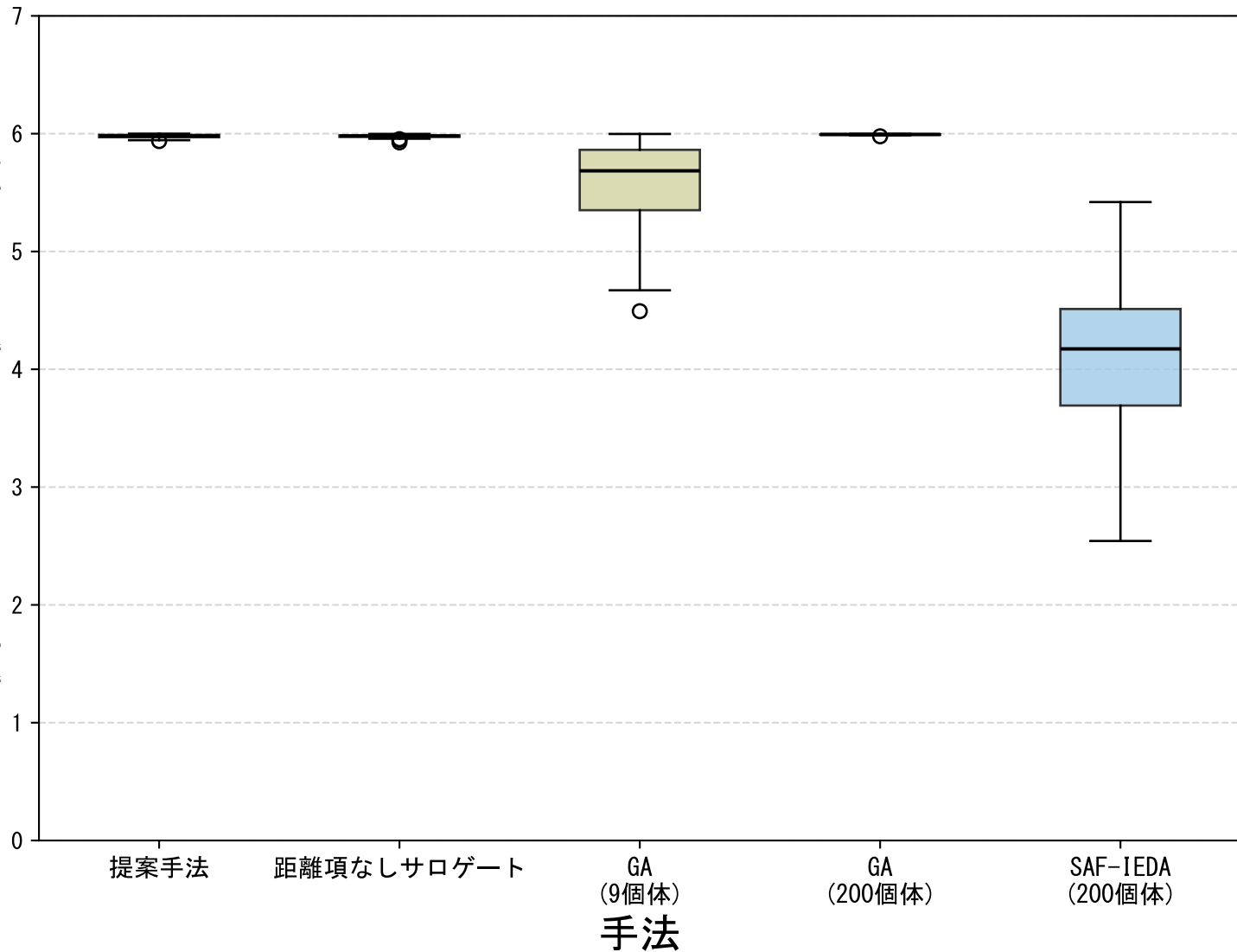
最終世代における最大適応度
