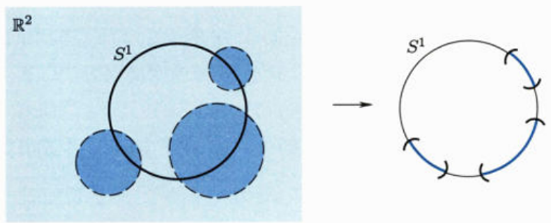
图 2.5: S^1 上的拓扑基
