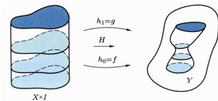
图 10.1: 同伦示意图
