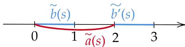
图 10.26: 道路连接
