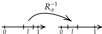
图 2.2: R_\alpha 保持测度
