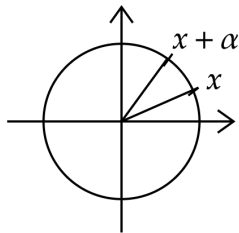
图 2.5: [0, 1) 表为圆周
