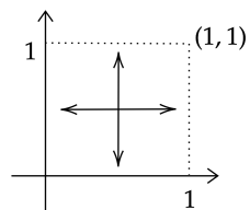
图 2.7: 二维环面
