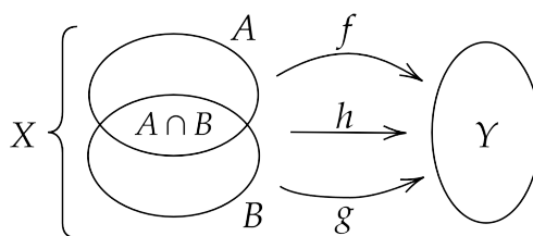
图 3.1: 粘贴引理示意图
